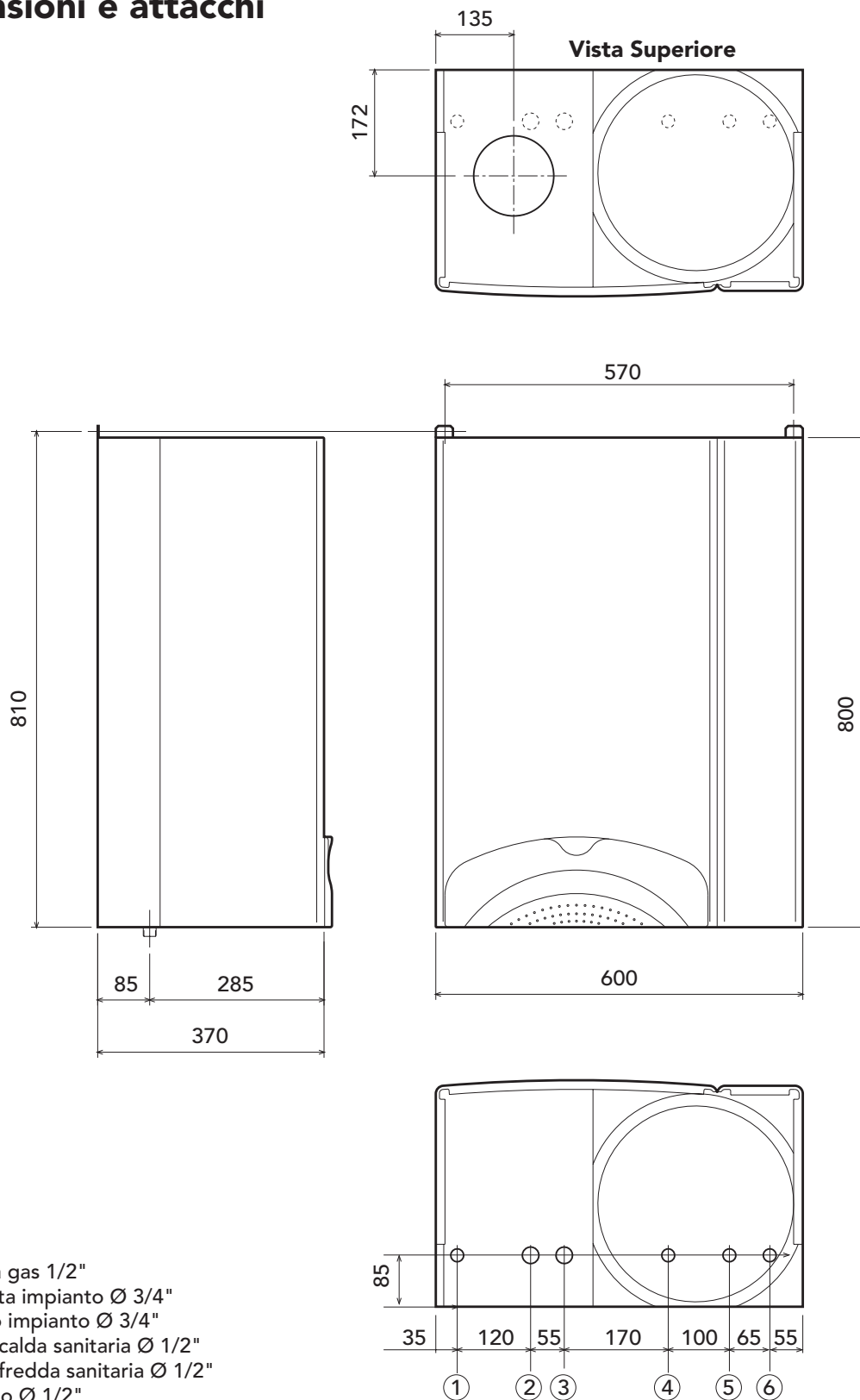
Vista Inferiore
