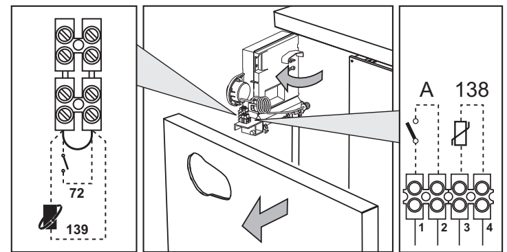
şek. 14 - Terminal kutusuna erişim
