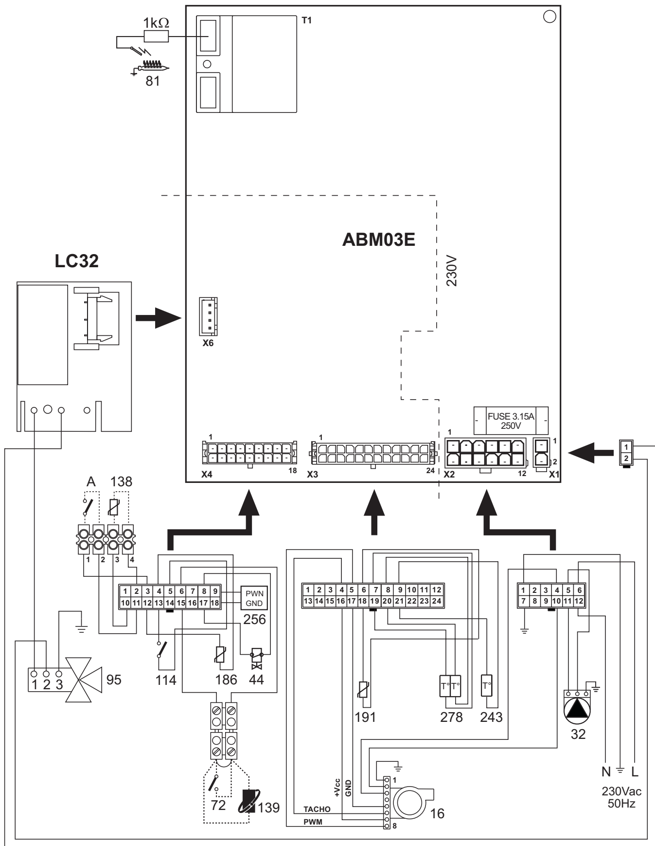
fig. 31 - Schéma électrique
