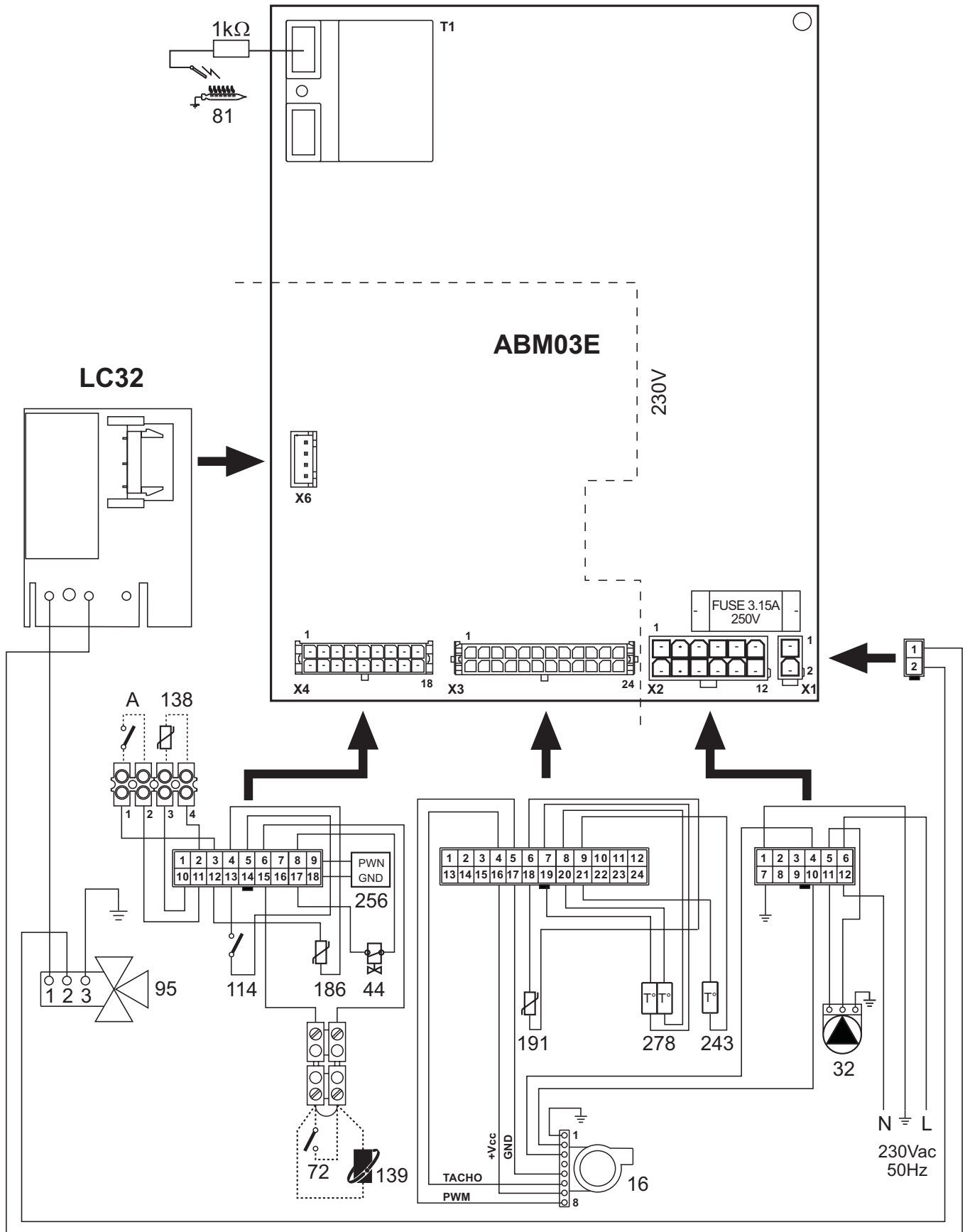
fig. 31 - Wiring diagram
