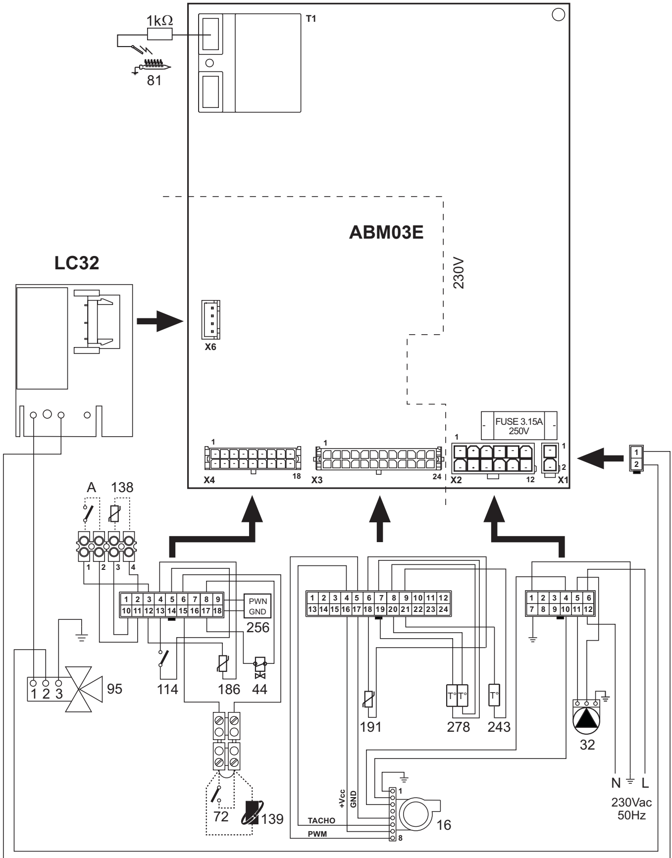
fig. 31 - Schema elettrico
