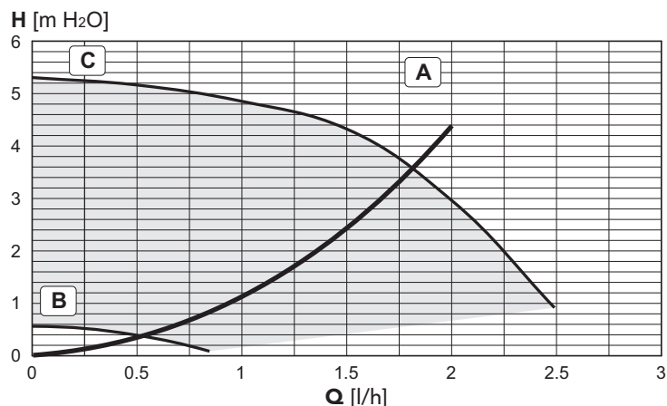
fig. 30 - Pertes de charge/pression circulateur BLUEHELIX B 32 K 50
