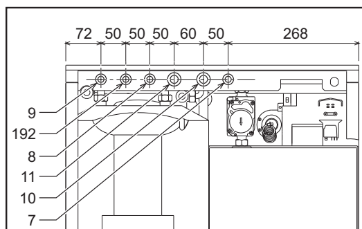
рис. 13 - Гидравлические штуцеры
