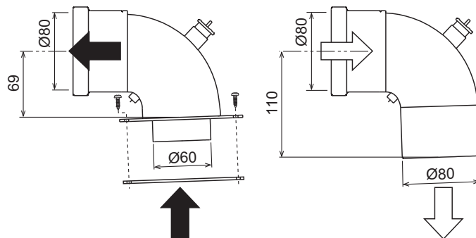
fig. 18 - Accesorio inicial para conductos separados
