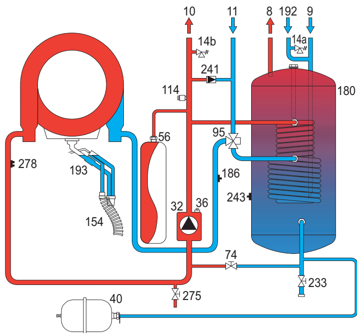
fig. 29 - Circuito hidráulico
