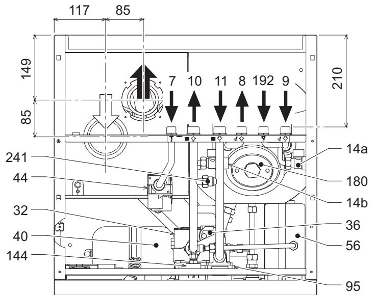
fig. 28 - Vista dall'alto (INGRESSO ARIA = □ / USCITA FUMI = ■)
