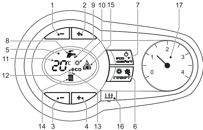
рис. 1 - Панель управления
