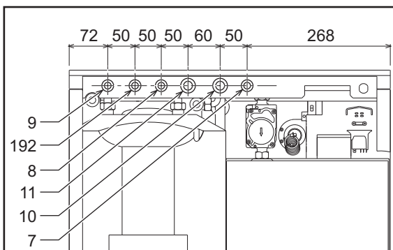
fig. 13 - Attacchi idraulici
