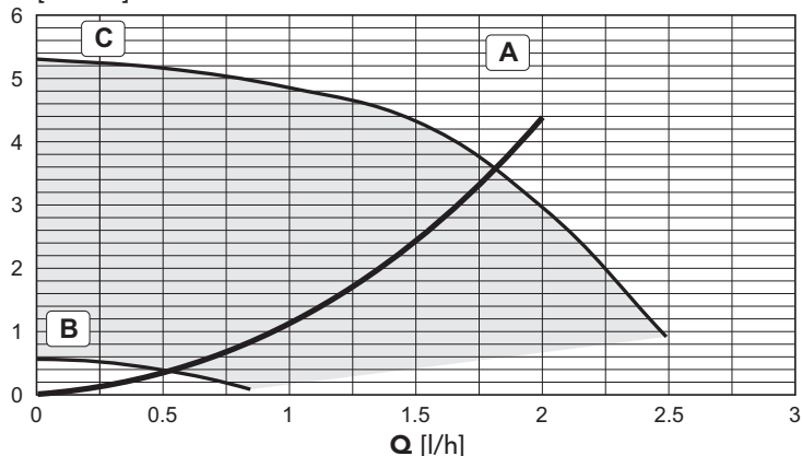
мал. 30 - Втрати напору / Напір циркуляційних насосів BLUEHELIX B 32 K 50
