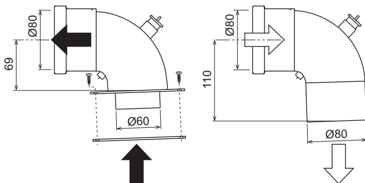
fig. 18 - Accessorio di partenza per condotti separati
