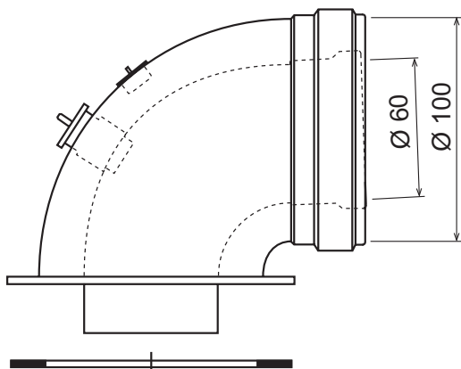
fig. 16 - Accessori di partenza per condotti coassiali
