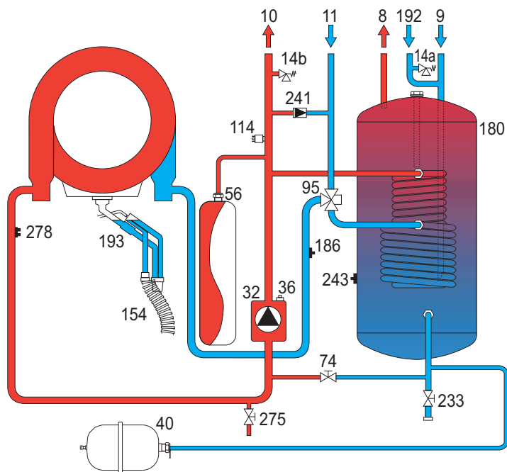
fig. 29 - Circuit hydraulique
