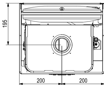
VISTA SUPERIORE
