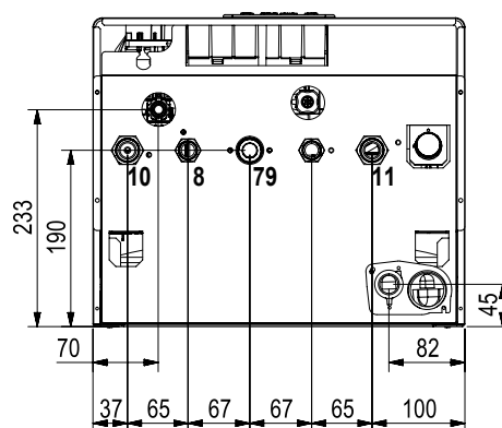
VISTA INFERIORE
