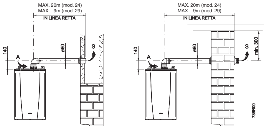
KIT FUMI PER ESTERNI
