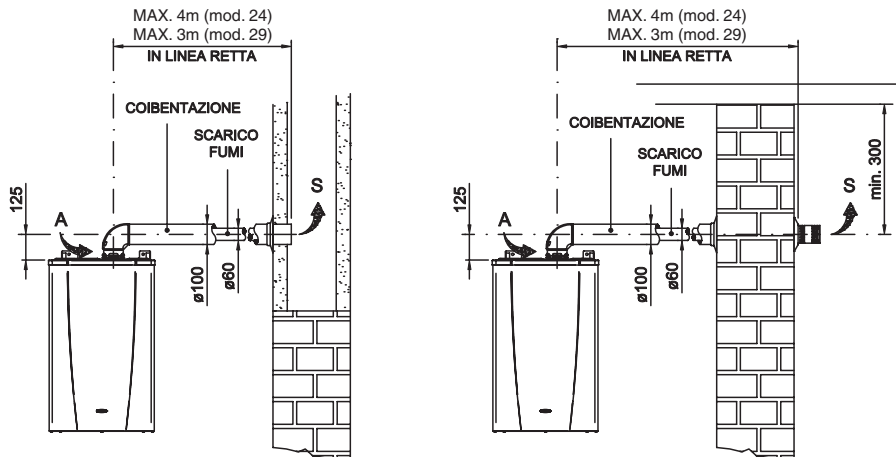
KIT FUMI PER ESTERNI COIBENTATO
