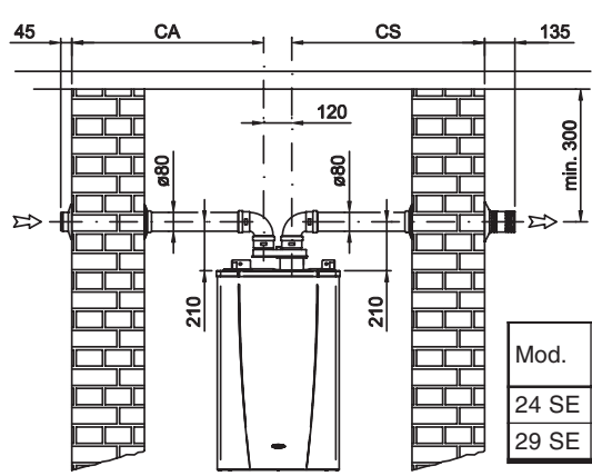
KIT FUMI SDOPPIATO ORIZZONTALE (Esempio N° 1, 2, 3)
