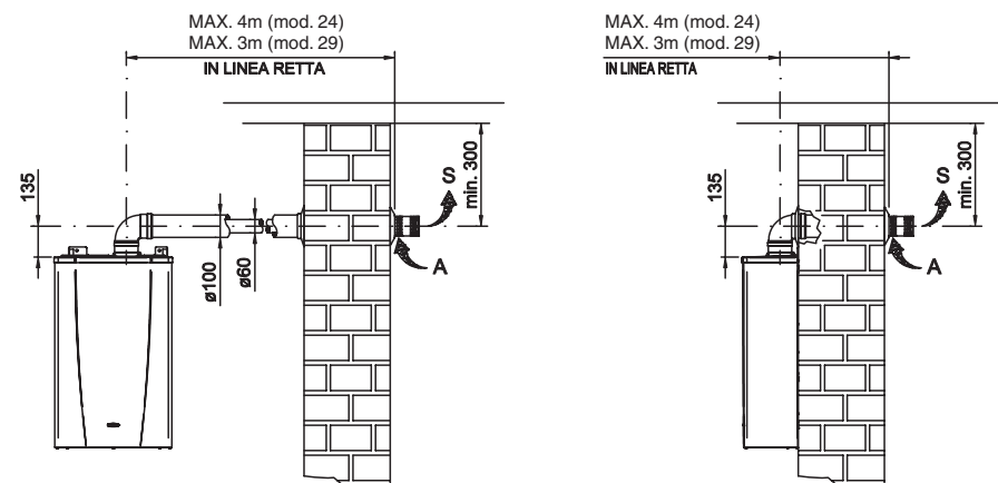
KIT FUMI COASSIALE ORIZZONTALE
