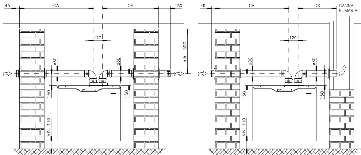
ASPIRAZIONE E SCARICO IN PARETE
