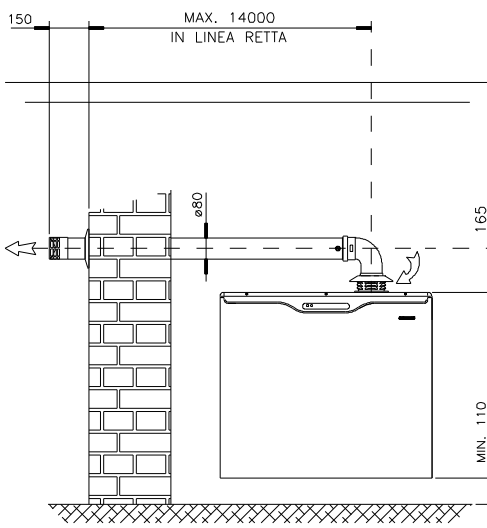
SCARICO A PARETE O DIRETTAMENTE ALL'ESTERNO E ASPIRAZIONE ALL'ESTERNO
