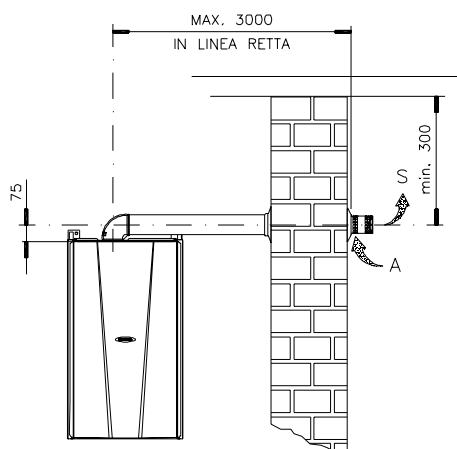
KIT FUMI COASSIALE ORIZZONTALE
