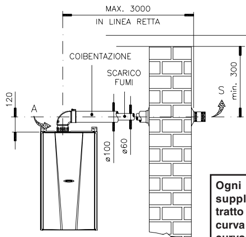
KIT FUMI PER ESTERNI COIBENTATO
