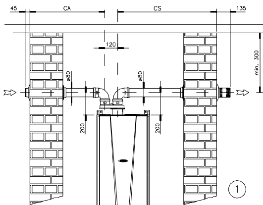
KIT FUMI SDOPPIATO ORIZZONTALE (Esempio N° 1, 2, 3)
