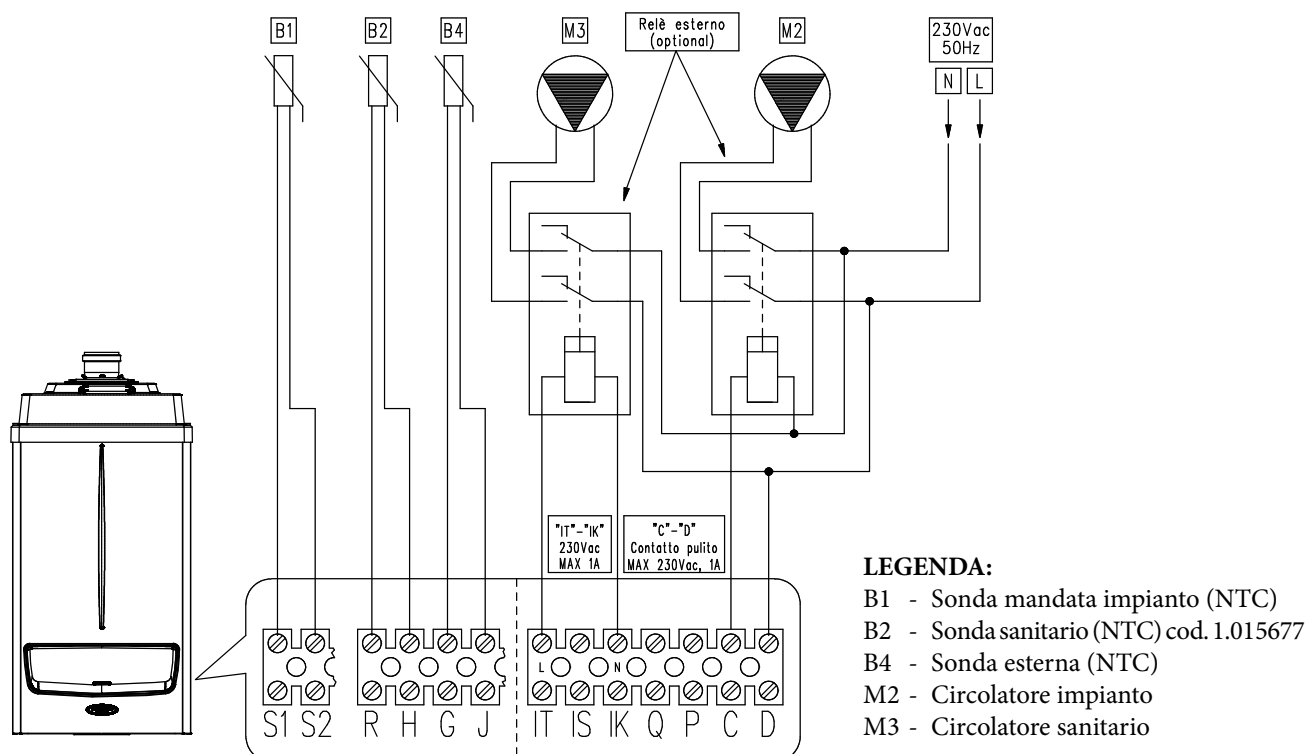
Schema elettrico di collegamento sonde e circolatori
