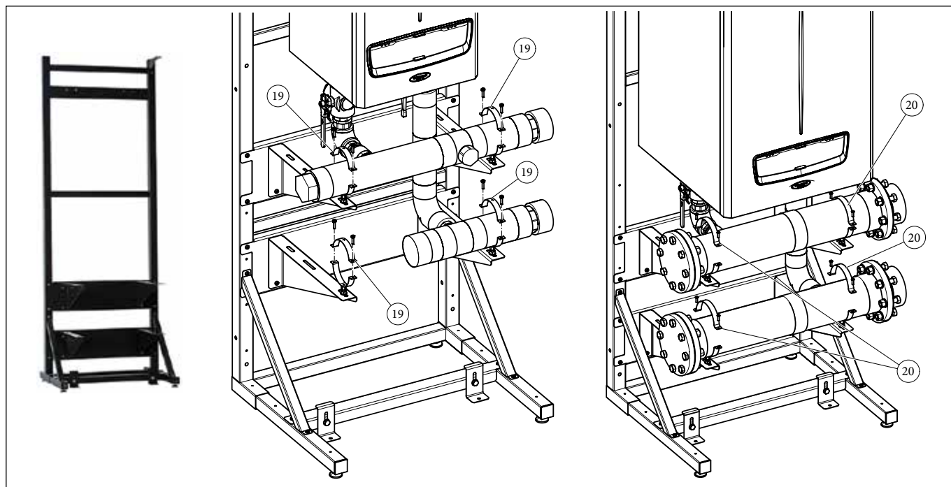
VICTRIX PRO 35 - 55
