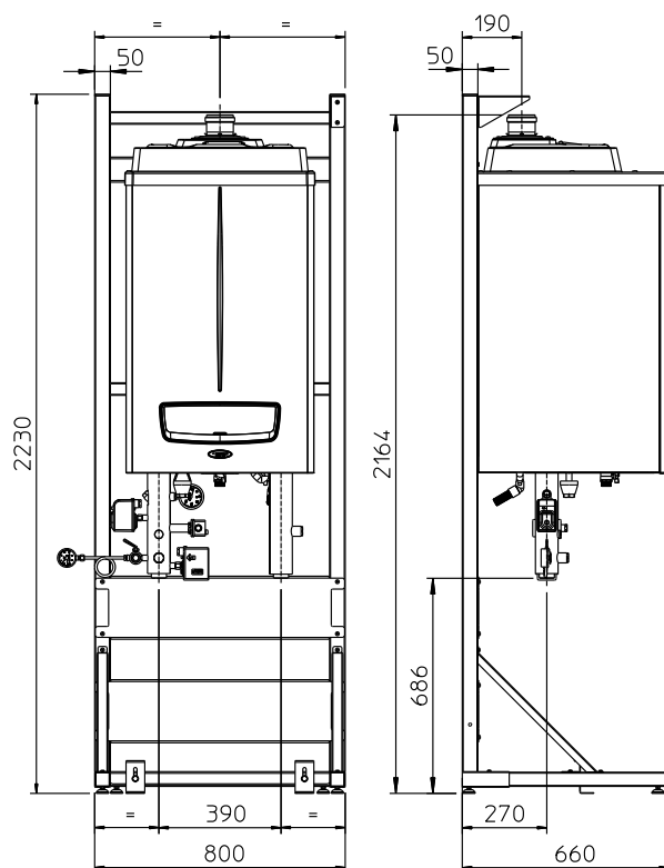
VICTRIX PRO 80 - 100 - 120
