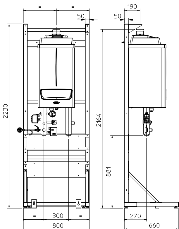
VICTRIX PRO 35 - 55
