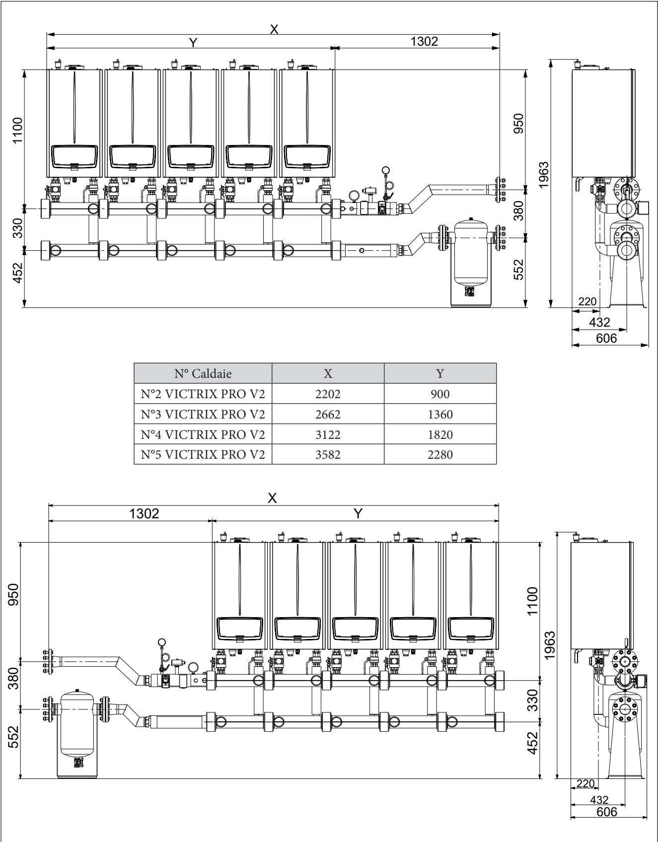
21.3 DIMENSIONI ED ATTACCHI CON KIT DEFANGATORE A DX / SX PER INSTALLAZIONE IN BATTERIA VICTRIX PRO 35 - 55 - 80 V2 (COD: 3.033674) (FINO AD UN MASSIMO DI CINQUE APPARECCHI)
