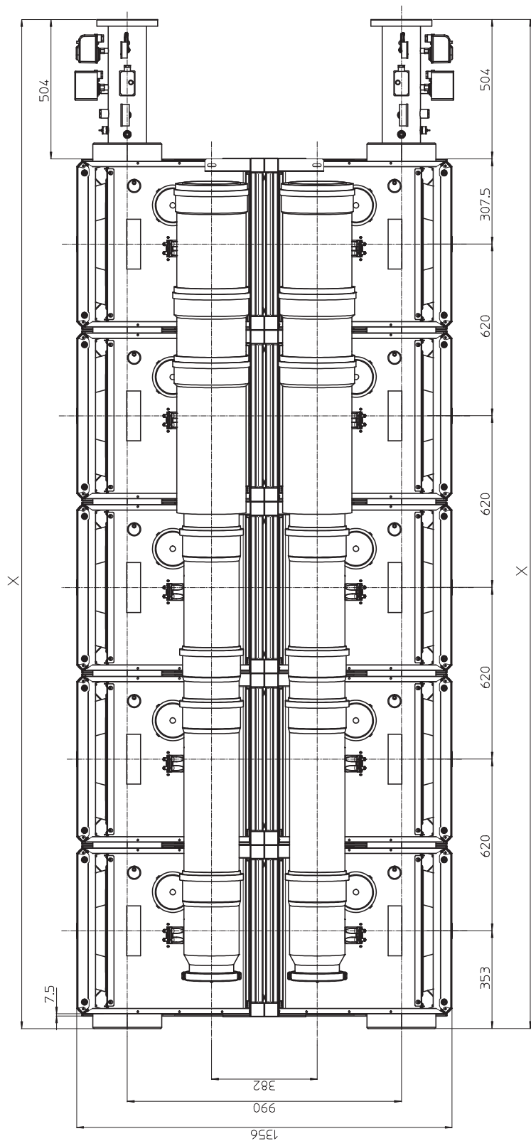
23.4 DIMENSIONI ED ATTACCHI CON KIT (OPTIONAL) VICTRIX PRO 150 V2 CON INSTALLAZIONE SU TELAIO DI SOSTEGNO POSTO SCHIENA CONTRO SCHIENA (FINO AD UN MASSIMO DI CINQUE APPARECCHI IN LINEA CON UNICO KIT INAIL)
