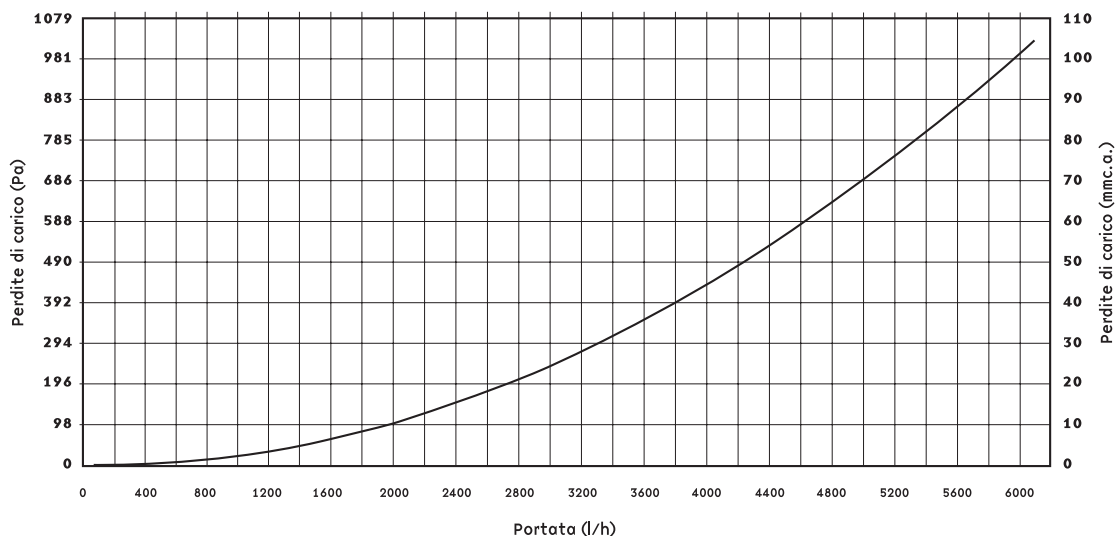
Grafico perdite di carico filtro raccolta fanghi
