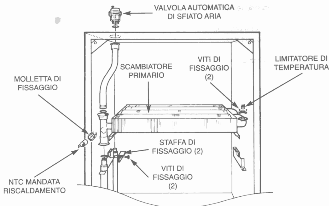
Fig. 20: Scambiatore principale
