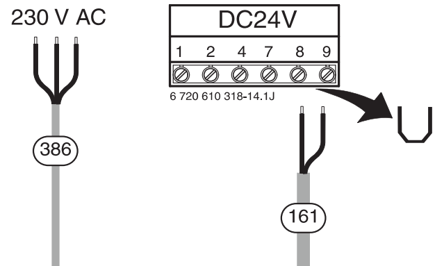
Fig. 20 Eliminare il collegamento con la Bosch Heatronic – ponticello 8-9!
