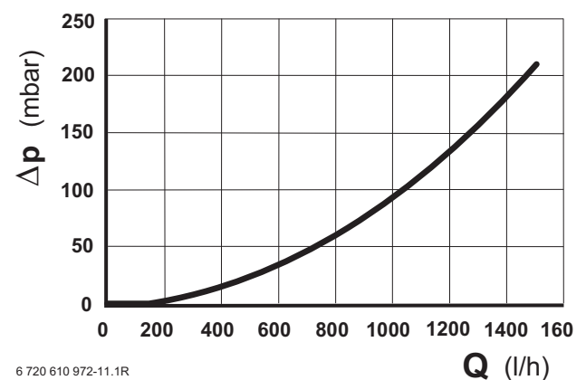
Fig. 11 Perdite di carico per apparecchi di tipo KBR
