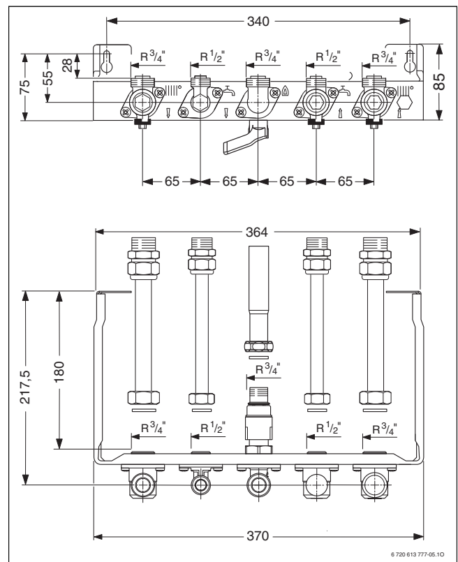
Fig. 8 Tubazioni a vista, realizzate in rame con brasatura piastra d'installazione, acc. nr. 893/18
