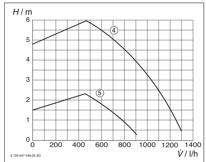
Fig. 38 Pressione proporzionale
