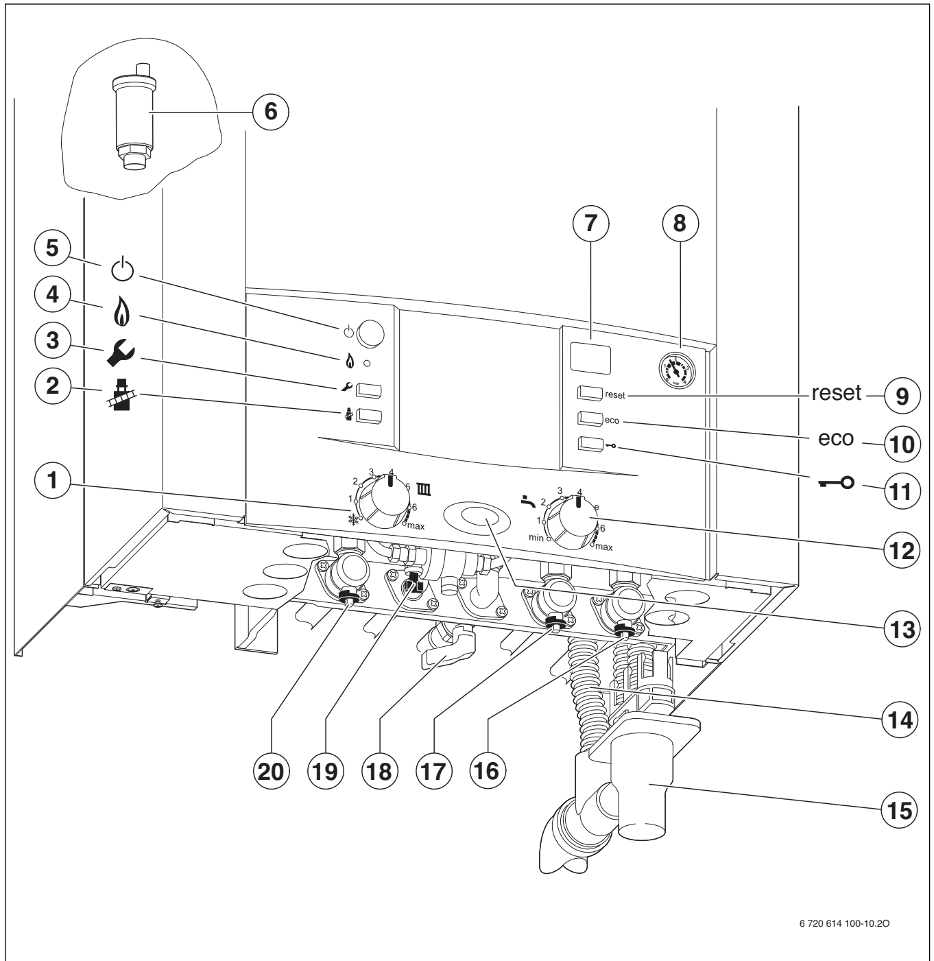
Fig. 25 Vista caldaia con accessorio nr. 893/18
