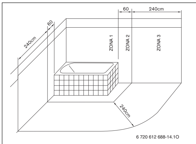
Fig. 19 Raffigurazione della Zona 3 (CEI 64-8)
