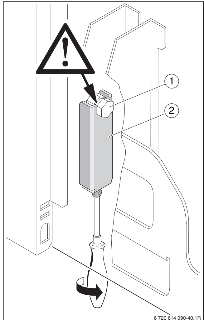
Fig. 12 Chiudere il fermo
