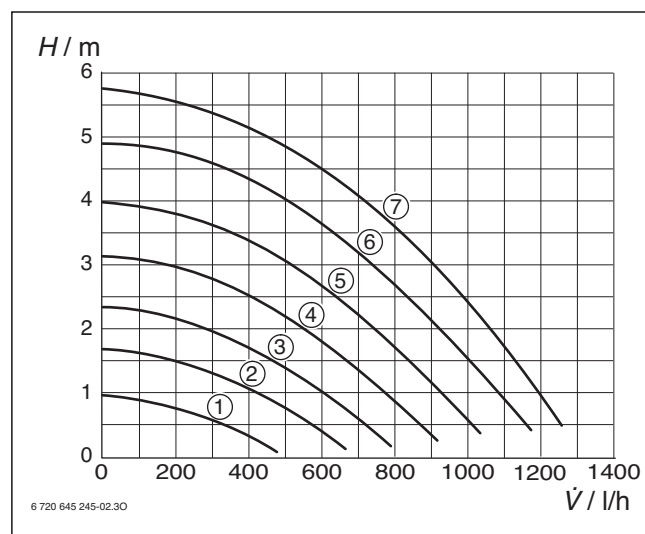
Fig. 39 Curve caratteristiche del circolatore
