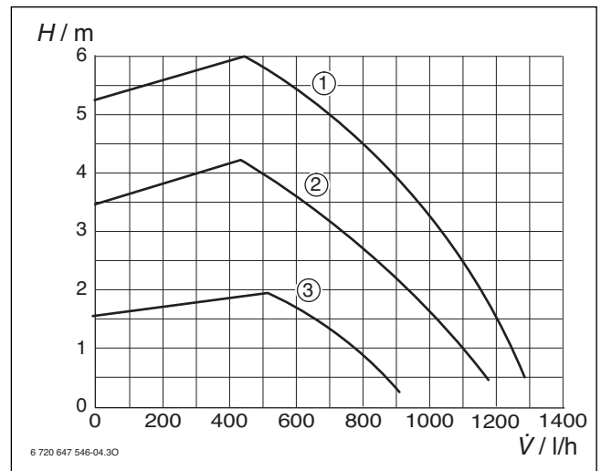
Fig. 37 Pressione costante
