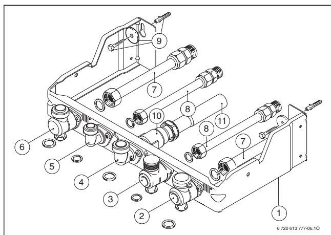
Fig. 9 Piastra d'intallazione, accessorio nr. 893/18
