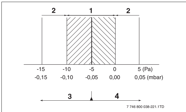
Fig. 42 Intervallo di impostazione della pressione differenziale in caso di carico parziale
