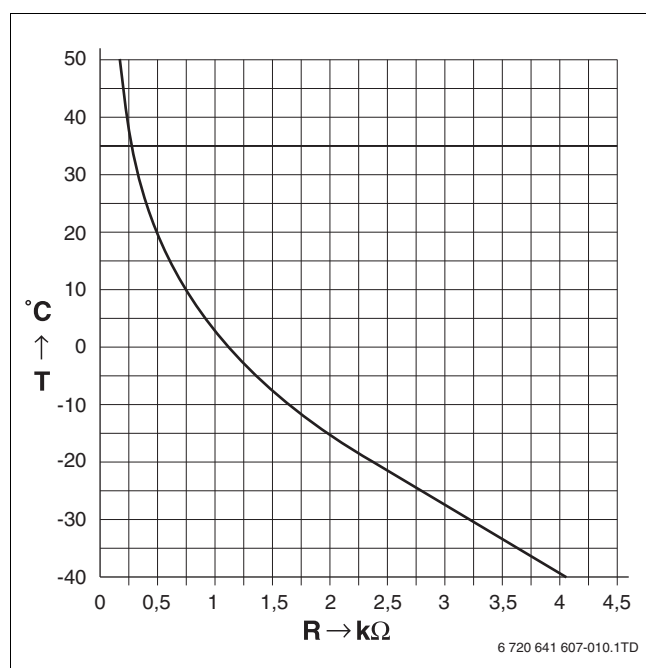
Fig. 84 Linea caratteristiche dalla resistenza della sonda della temperatura esterna
