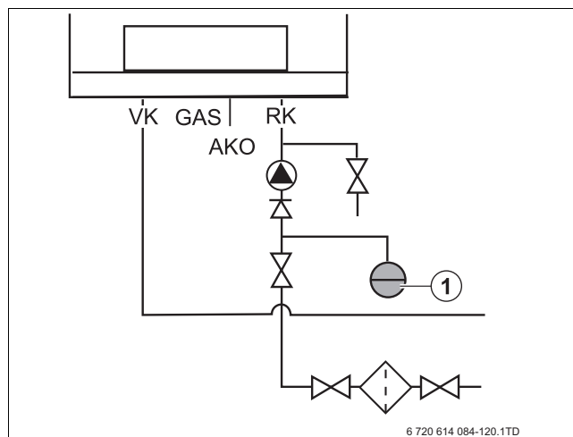
Fig. 16 Collegamento vaso di espansione senza compensatore idraulico
