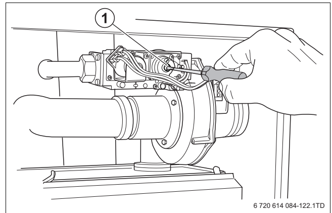
Fig. 43 ZBR 98-2: vite di regolazione rapporto gas-aria
