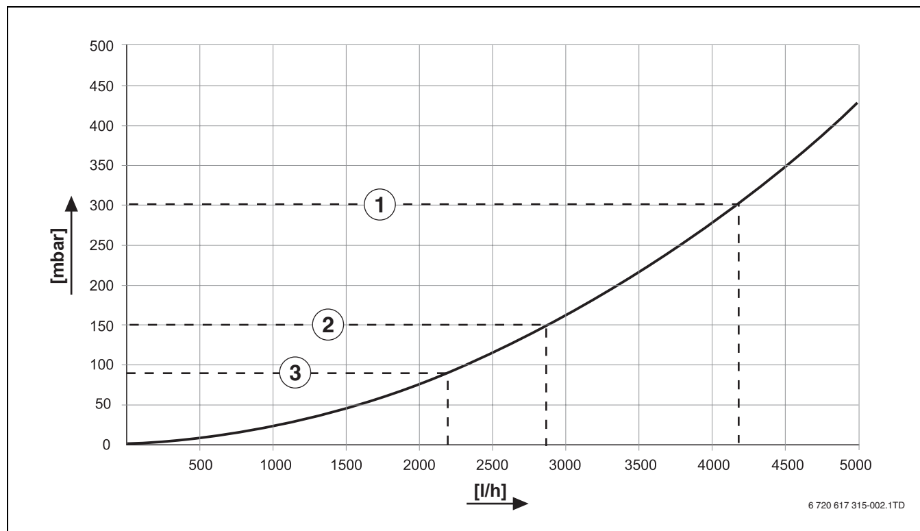
Fig. 83 Linea caratteristiche dalla resistenza
