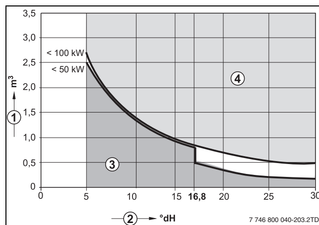
Fig. 6 Requisiti dell'acqua di riempimento della caldaia per caldaia singola fino a 100 kW
