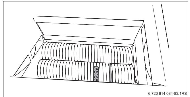
Fig. 65 Verifica del dispositivo di accensione a incandescenza e dell'elettrodo d'ionizzazione
