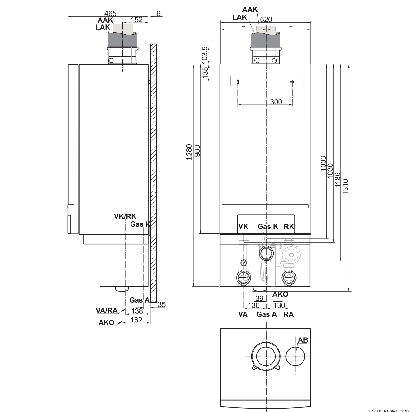
Fig. 3 Dimensioni e collegamenti con gruppo di collegamento [mm]
