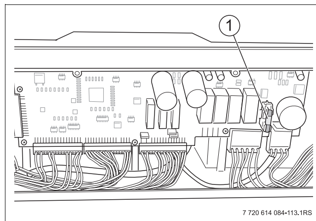
Fig. 79 Fusibile
