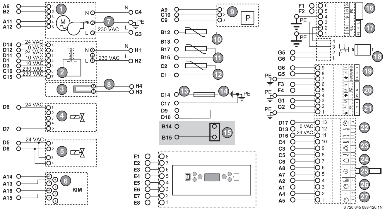
Fig. 5 Schema dei collegamenti
