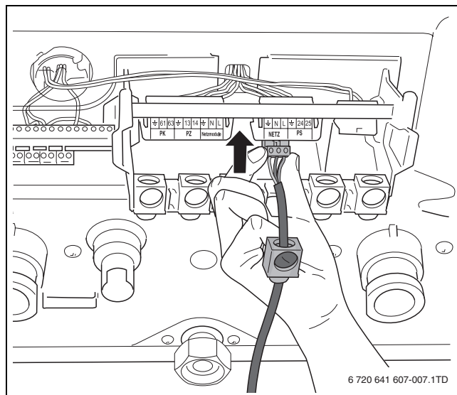
Fig. 22 Inserimento connettore
