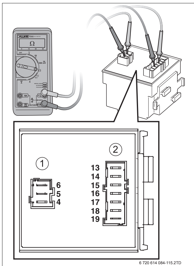
Fig. 81 Controllo trasformatore
