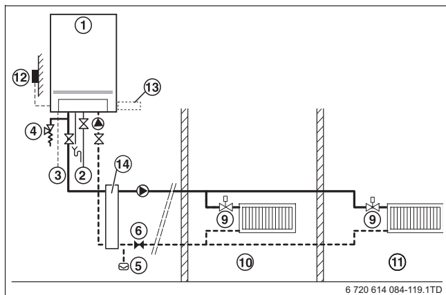
Fig. 8 Esempi di applicazione con regolazione climatica
