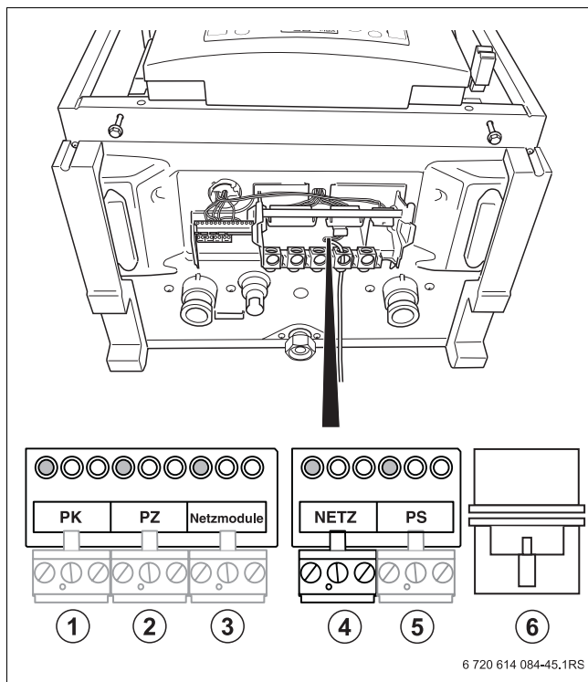
Fig. 21 Morsettiera cavi
