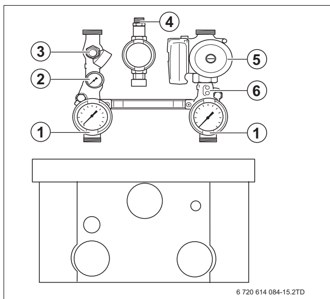
Fig. 10 Gruppo di collegamento
