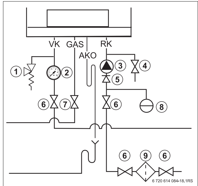
Fig. 12 Collegamenti lato acqua e lato gas
