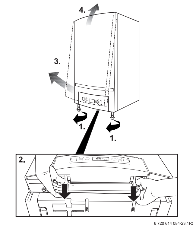
Fig. 18 Smontaggio copertura caldaia pannello anteriore
