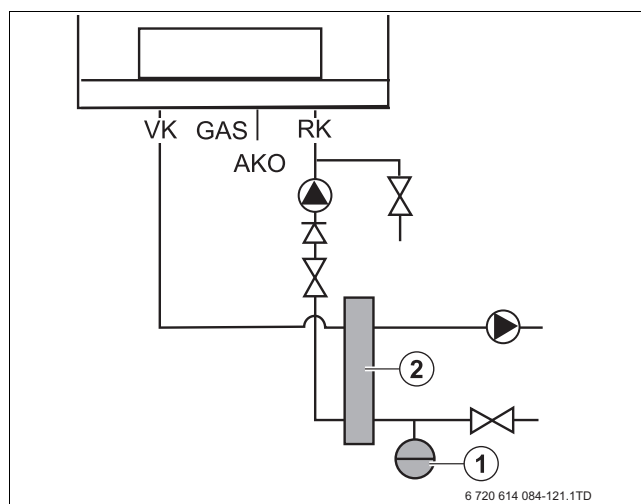
Fig. 17 Collegamento vaso di espansione con compensatore idraulico
