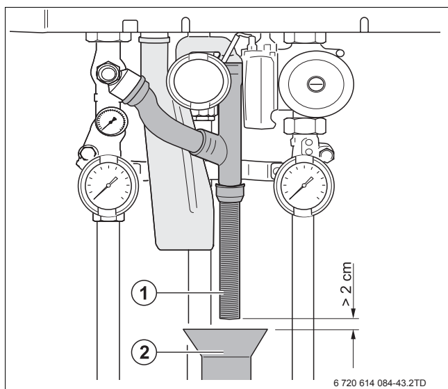
Fig. 15 Distanza minima dal tubo ondolato
