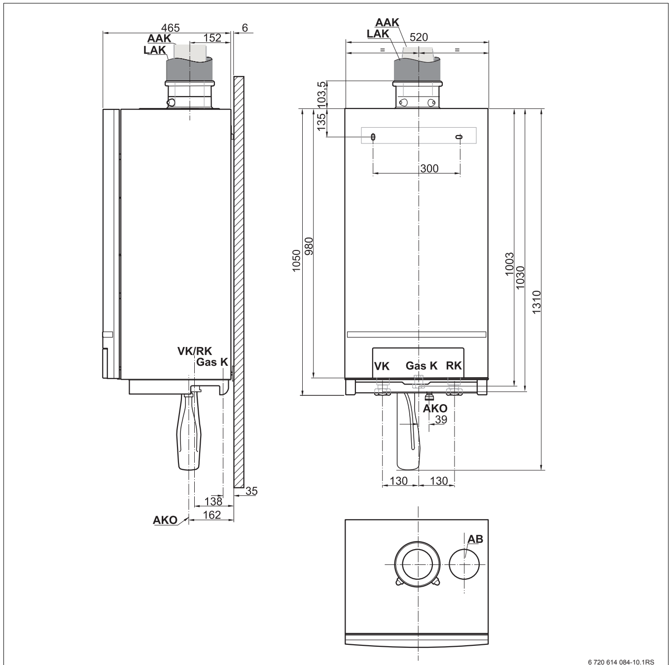
Fig. 2 Dimensioni e collegamenti senza gruppo di collegamento [mm]
