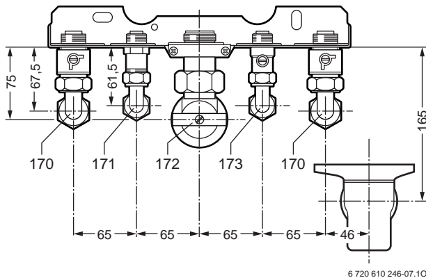
Fig. 8 Piastra di allacciamento (installata)
