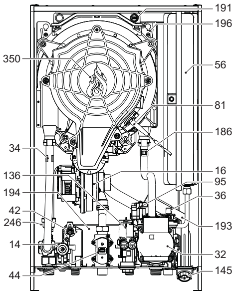
fig. 76- Vedere generală
