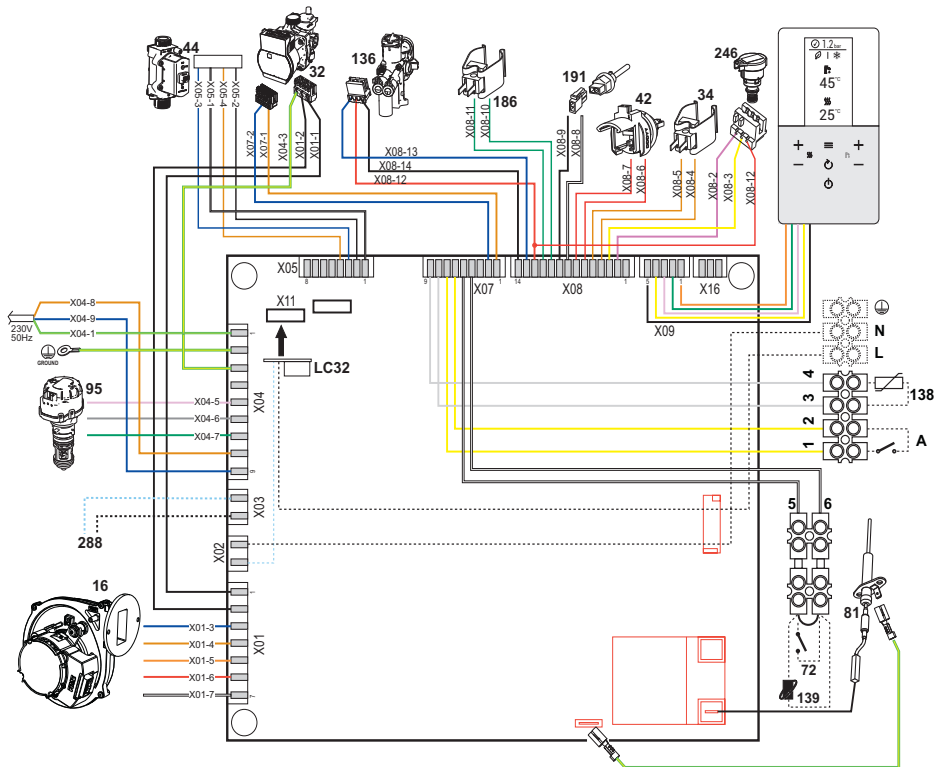
fig. 80- Wiring diagram
