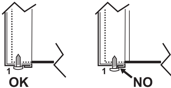
fig. 57 - Posizione corretta pannello frontale
