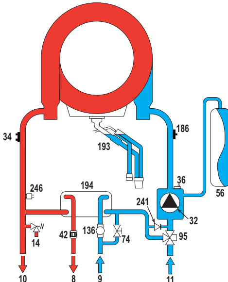
fig. 77- Circuitul hidraulic
