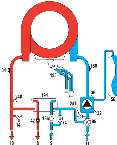
wygląd 77- Obieg wody
