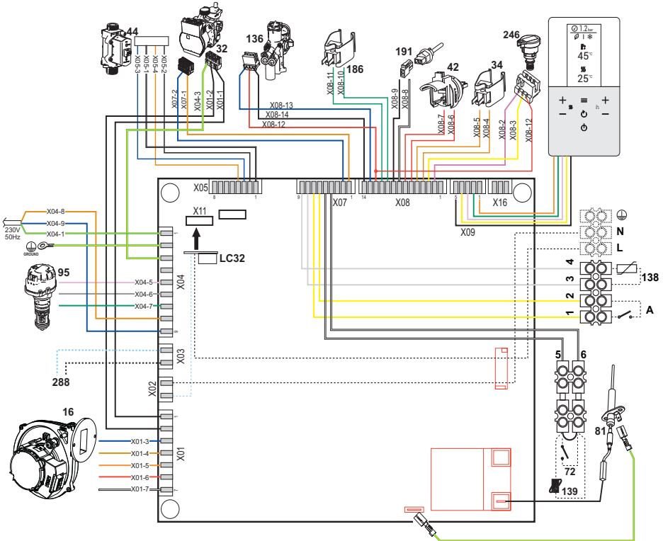
fig. 80 - Esquema eléctrico
