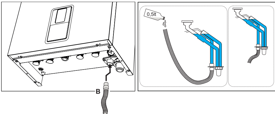
fig. 52 - Collegamento scarico condensa
