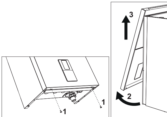
εικ. 41- Άνοιγμα μπροστινού πίνακα
