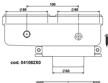
wygląd 36- Człon początkowy do montażu oddzielnych przewodów
