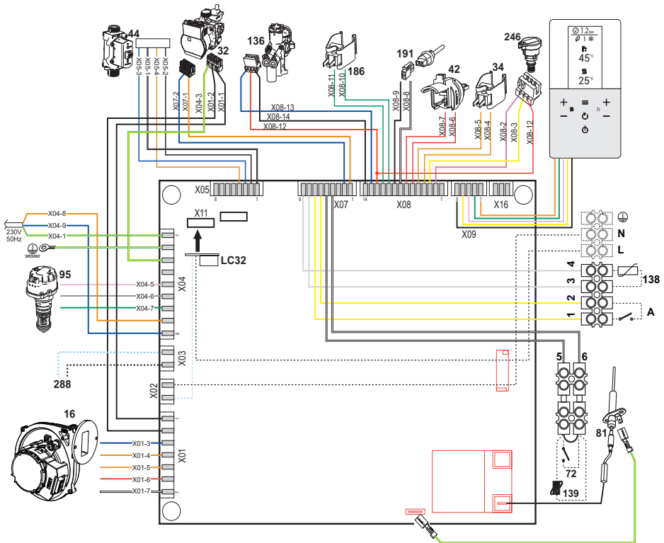
wygląd 80- Schemat instalacji elektrycznej
