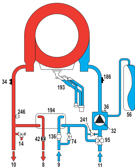
εικ. 63- Υδραυλικό κύκλωμα
