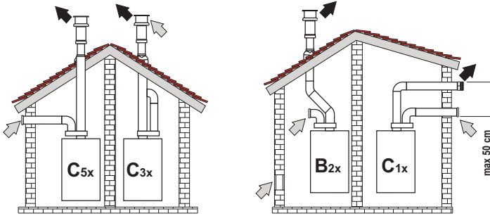
εικ. 33- Παραδείγματα σύνδεσης με ξεχωριστούς σωλήνες (⇨ = Αέρας / ⇨ = Καυσαέρια)
