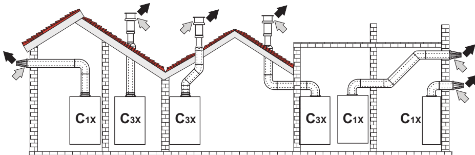
wygląd 31- Przykłady połączenia przewodami współosiowymi
