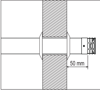
Distancia del terminal (tipo C13)
