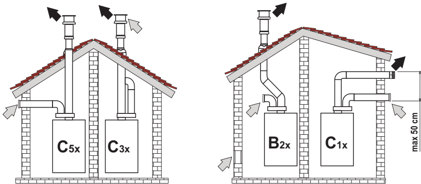
fig. 35 - Esempi di collegamento con tubi separati
