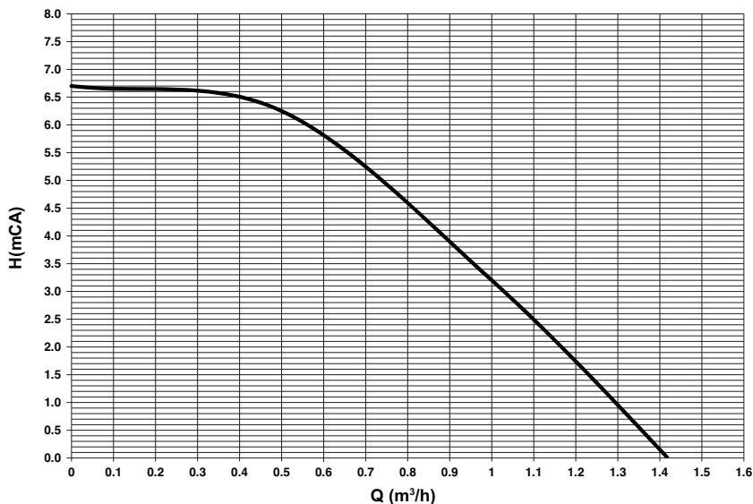
fig. 78- Înălțime de pompare reziduală disponibilă în instalație
