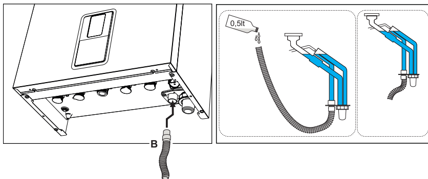
wygląd 52- Podłączenie spustu kondensatu
