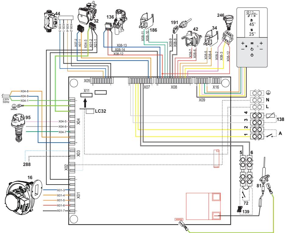
fig. 80 - Schema electrică
