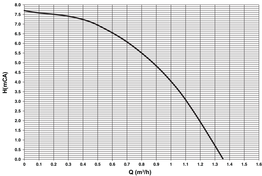
fig. 80 - Prevalenza residua disponibile all'impianto
