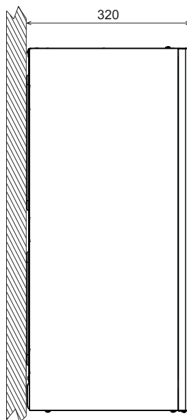
fig. 73- Vedere laterală
