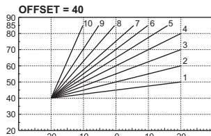
fig. 25- Exempu de deplasare paralelă a curbelor de compensare
