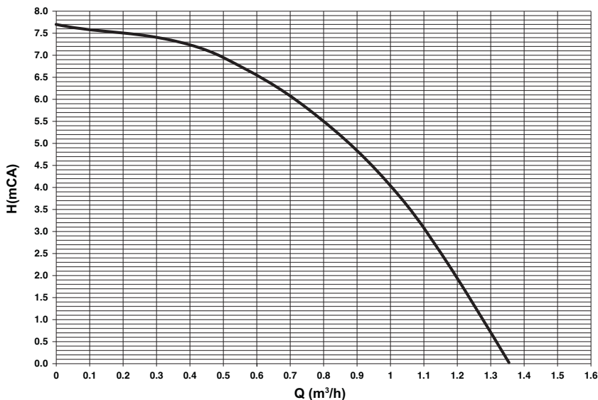
fig. 79- Înălțime de pompare reziduală disponibilă în instalație
