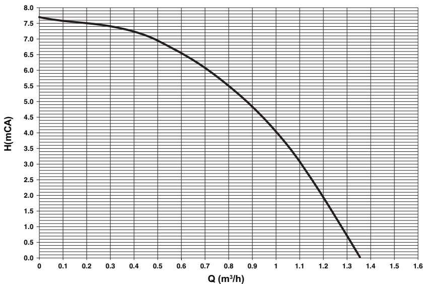
wygląd 79- Wysokość podnoszenia dostępna w instalacji
