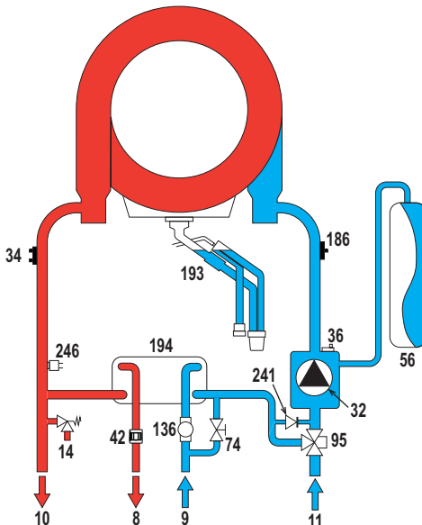
fig. 78 - Circuito idraulico
