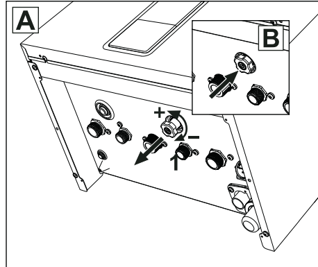
fig. 26 - Filling knob
