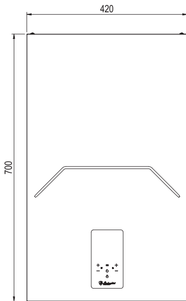
fig. 72- Vedere frontală
