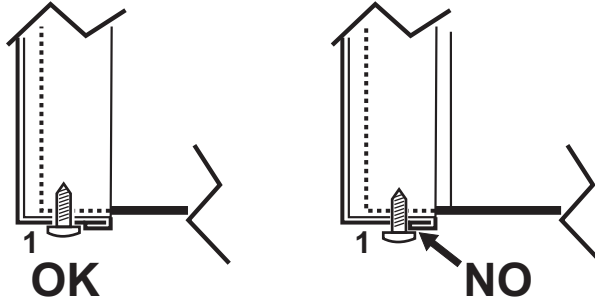
fig. 56- Posición correcta del panel frontal
