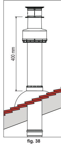
Distancia del terminal (tipo C33)
