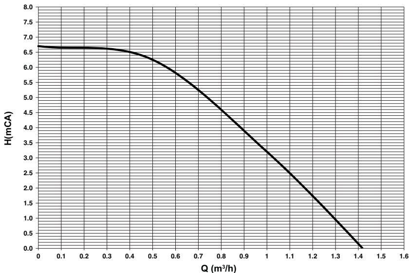
fig. 78- Carga hidrostática residual disponible en la instalación
