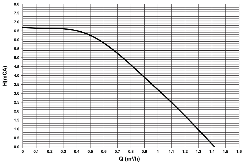
fig. 79 - Prevalenza residua disponibile all'impianto
