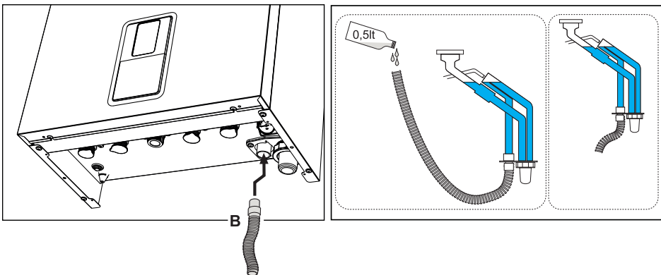
εικ. 38- Σύνδεση εξαγωγής συμπυκνώματος
