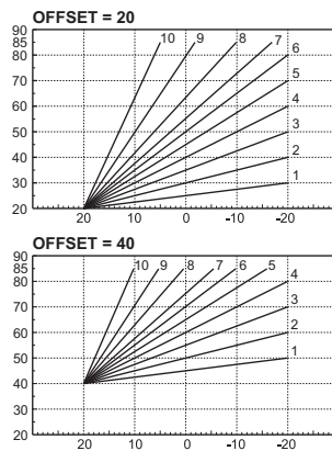
ΕΙΚ. 25- Παράδειγμα παράλληλης μετατόπισης των καμπυλών αντιστάθμισης
