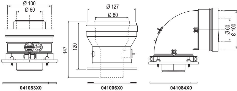
fig. 32- Accesorios iniciales para conductos coaxiales
