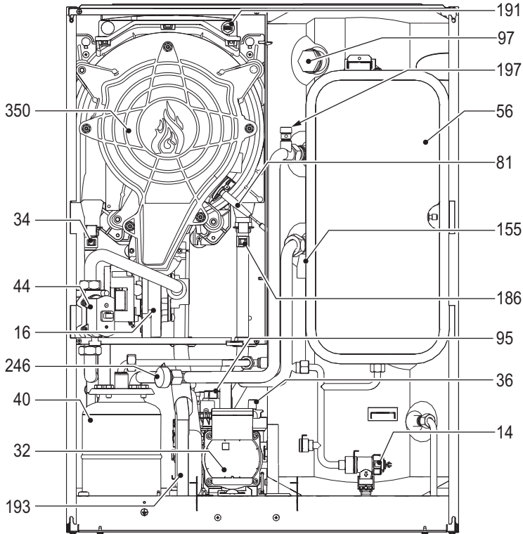
fig. 47 - Vista generale
