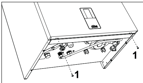
wygląd 41- Otwieranie panelu przedniego
