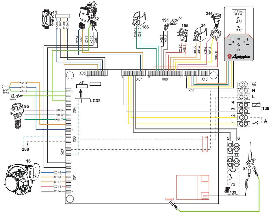
fig. 51- Schema electrică
