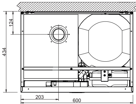
fig. 45- Vista superior
