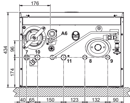
fig. 46- Vista inferior
