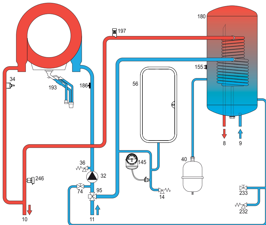
fig. 48- Circuitul hidraulic
