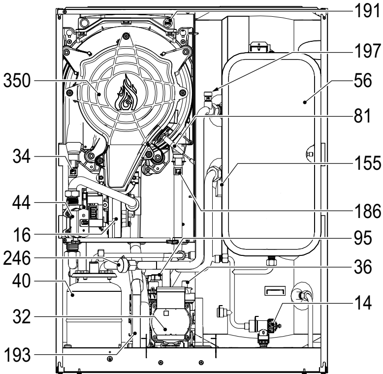
fig. 47 - Vista generale
