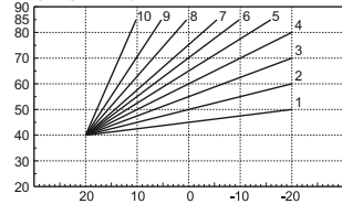
OFFSET = 40 fig. 25 - Esempio di spostamento parallelo delle curve di compensazione
