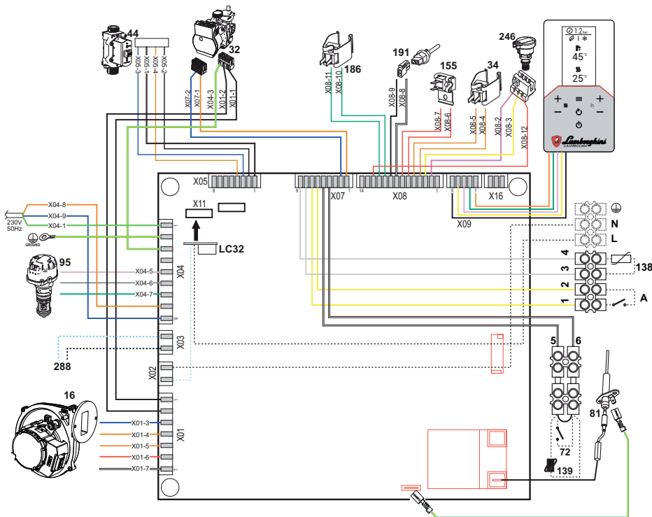
fig. 51- Esquema eléctrico
