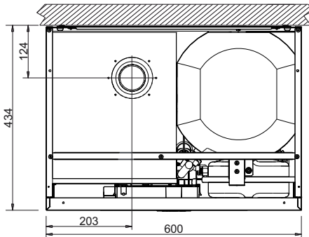
fig. 45- Vista superior
