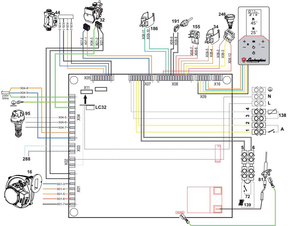
fig. 51 - Schema elettrico
