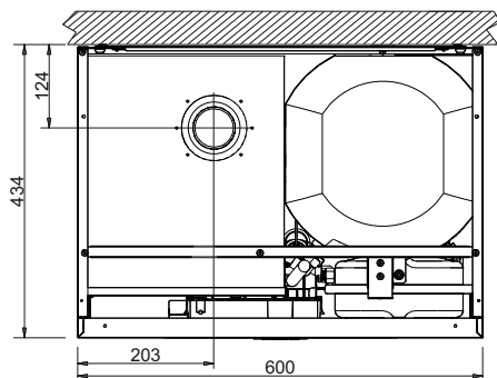
fig. 45 - Vista dall'alto
