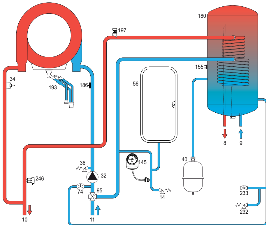
fig. 48 - Circuito idraulico
