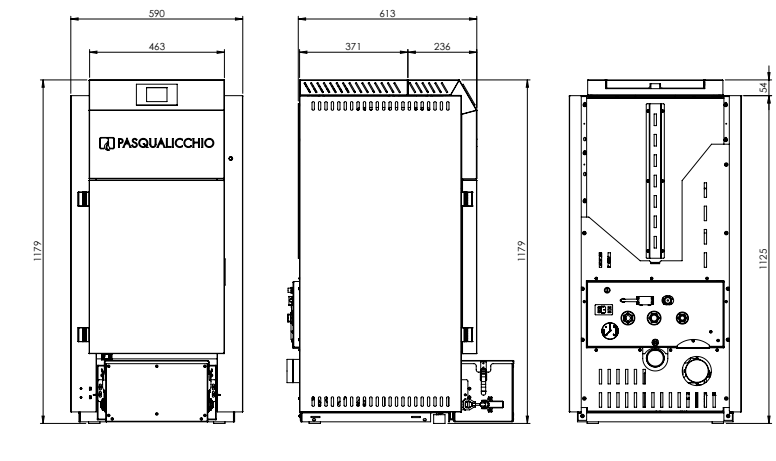
Cantinola Touch 18 con compattatore
