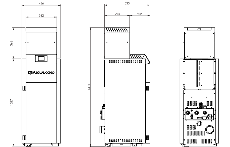
Cantinola Touch 15 con prolunga
