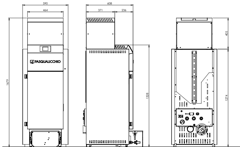
Cantinola Touch 24 - 29 con prolunga e compattatore
