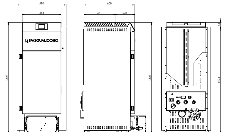
Cantinola Touch 24-29 kW con compattatore
