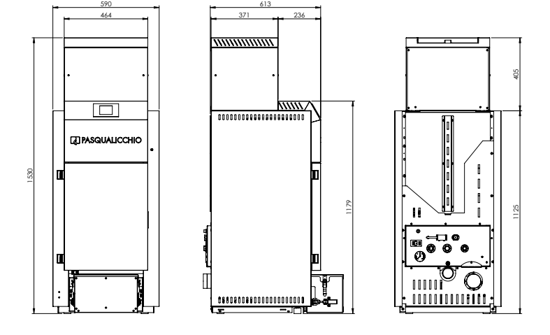
Cantinola Touch 18 con compattatore e prolunga
