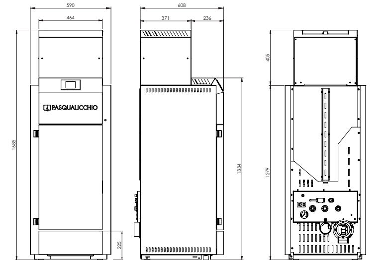
Cantinola Touch 24-29kW con prolunga
