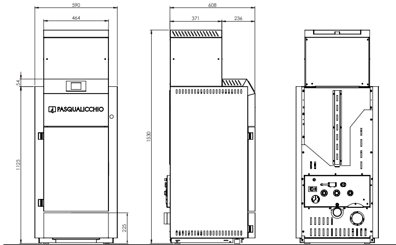
Cantinola Touch 18 con prolunga
