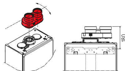
Kit sistema sdoppiato (da Ø60-100 a Ø80-80 mm) con ingresso aria a posizione variabile
