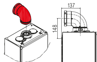
Condotto coassiale Ø60-100 mm
