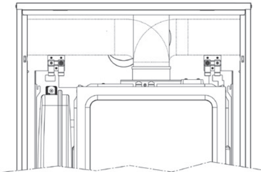
Condotti coassiali (ø 60-100mm)
