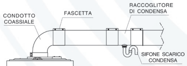
Condotti coassiali (ø 60-100mm)
