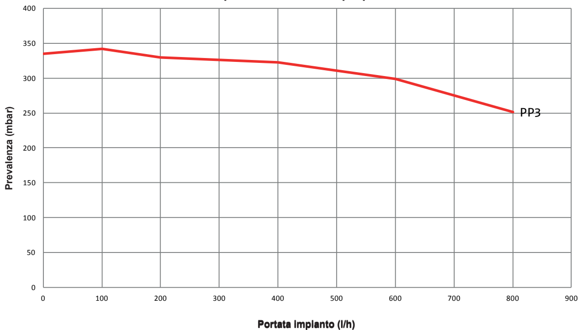
Curva prevalenza residua proporzionale
