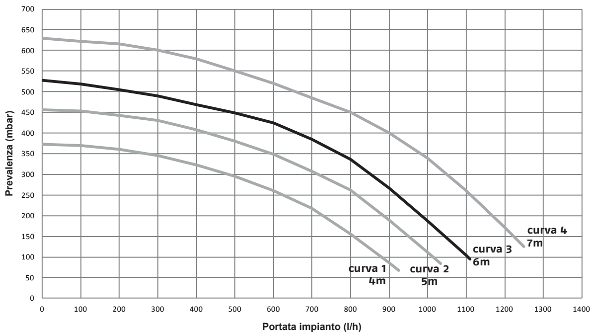
Curva prevalenza residua costante
