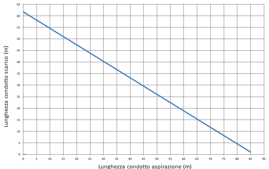
Residence Condens 32 IS i Lunghezza massima tubi \varnothing 80
