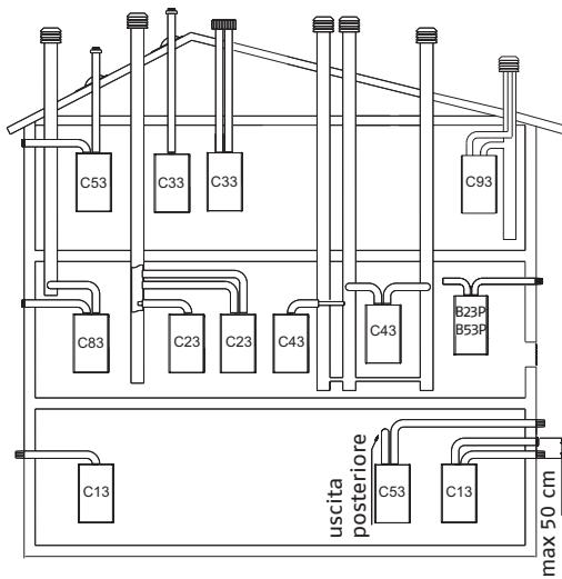
Residence Condens 20 IS i Lunghezza massima tubi \varnothing 80
