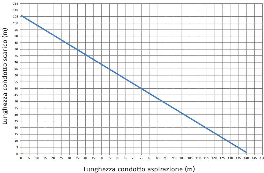
Residence Condens 32 IS i Lunghezza massima tubi \varnothing 80
