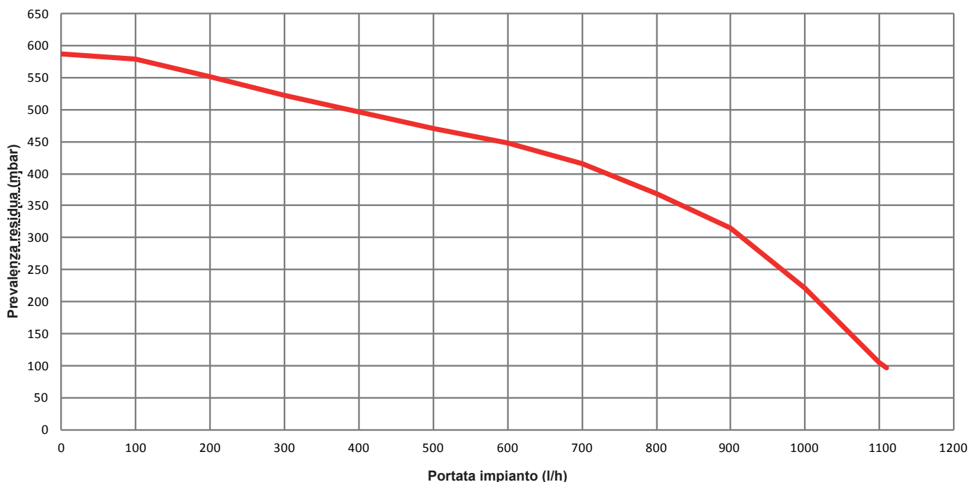
Grafico 2 (circolatore 7 metri)
