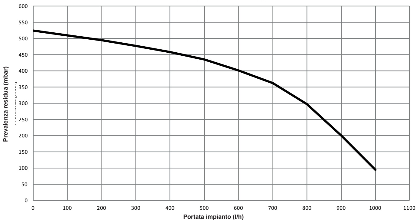
Grafico 1 (circolatore 6 metri)
