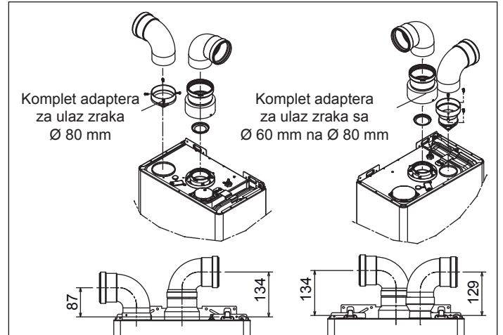
Maksimalna dužina cijevi Ø 80 mm - 25 IS
