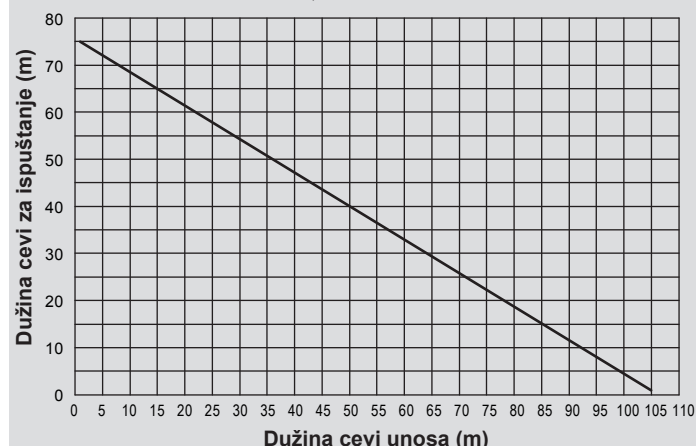
Maksimalna dužina cevi Ø 80 mm - 25 IS
