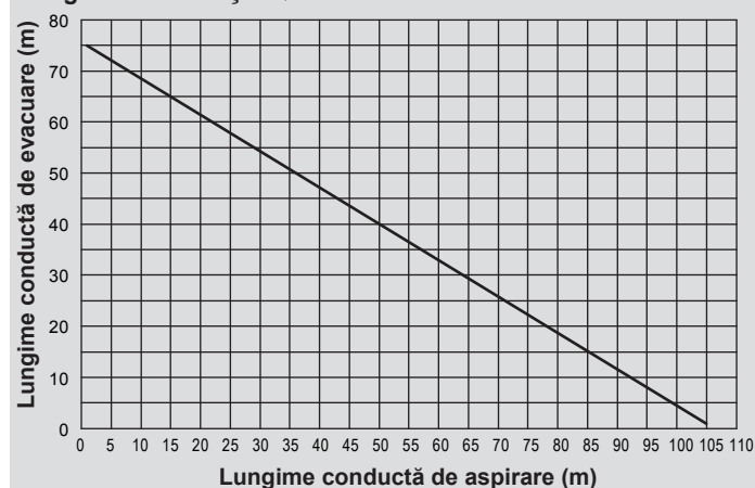
Lungime maximă țevi Ø 80 mm - 25 IS
