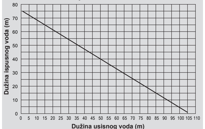
Maksimalna dužina cijevi Ø 80 mm - 25 IS
