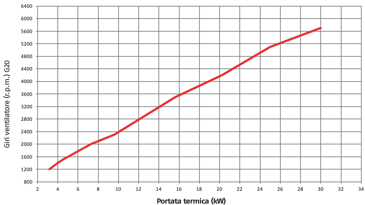
Curva portata termica - nr. giri ventilatore (MTN) - 3.0 KIS E
