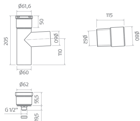
Raccordo a T \varnothing 60 mm con chiusura per scarico condensa
