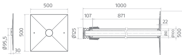
Collettore verticale \varnothing 60/100 mm con copertura camino
