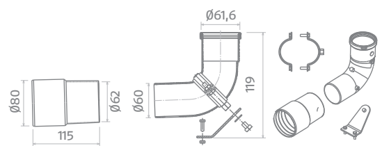
kit Collegamento camino 80-60 mm con curva 90° \varnothing 60 PP
