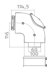
Curva 90° ispezionabile
