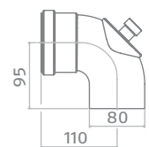
Curva 90° ispezionabile
