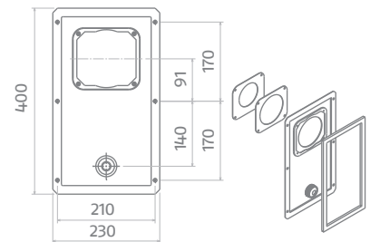
Kit pannello di chiusura per condotto fumi
