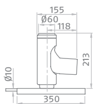
Kit supporto camino
