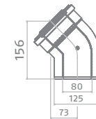
Curva 45°
