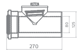
Tronchetto ispezione
