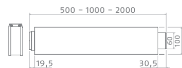
Tronchetto ispezione
