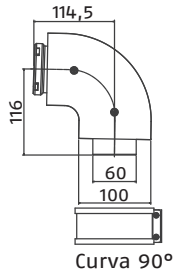
Curva 90°
