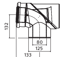
Curva 90°
