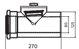
Tronchetto ispezione
