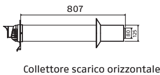
Collettore scarico orizzontale
