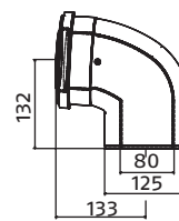
Curva 90°
