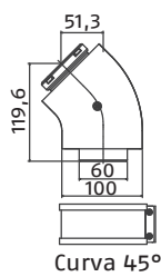
Curva 45°
