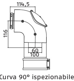
Curva 90°
