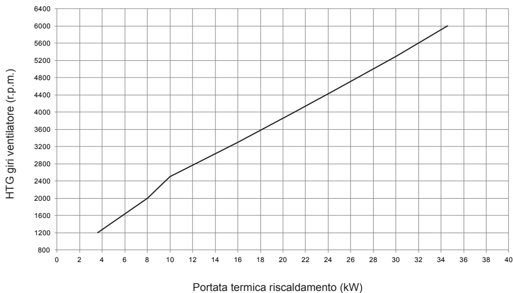
Curva portata termica - nr. giri ventilatore (Qnrisc) - 35 SR
