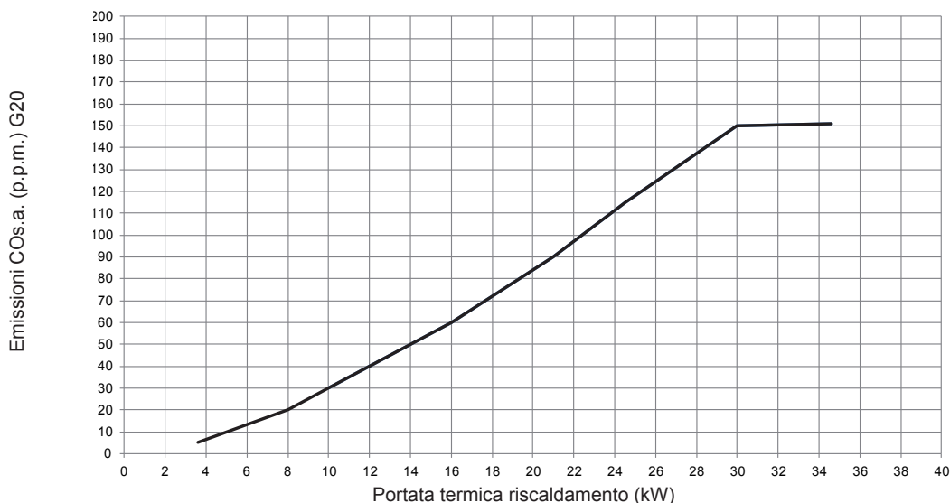
Curva portata termica - emissioni (Qnrisc) - 35 SR
