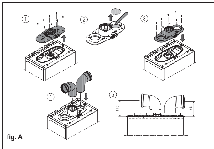
Sistema sdoppiato con utilizzo del kit collegamento sistema sdoppiato Ø80 (accessorio)
