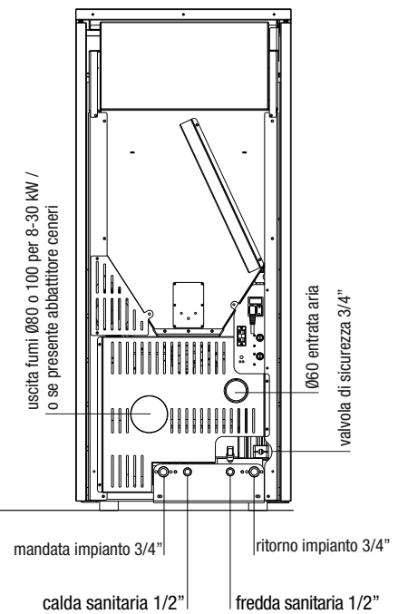
vista posteriore
