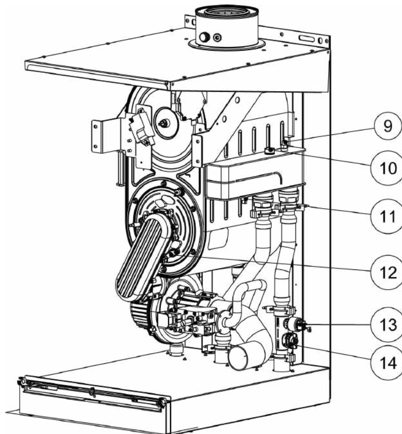
figura 3 - Componenti caldaia modelli da 80 a 115
