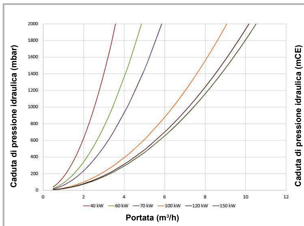
figura 17 - Cadute di pressione
