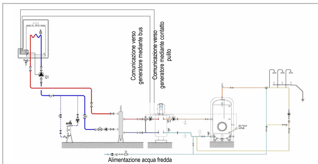
figura 36 - Schema VARFREE EVO22 Ter
