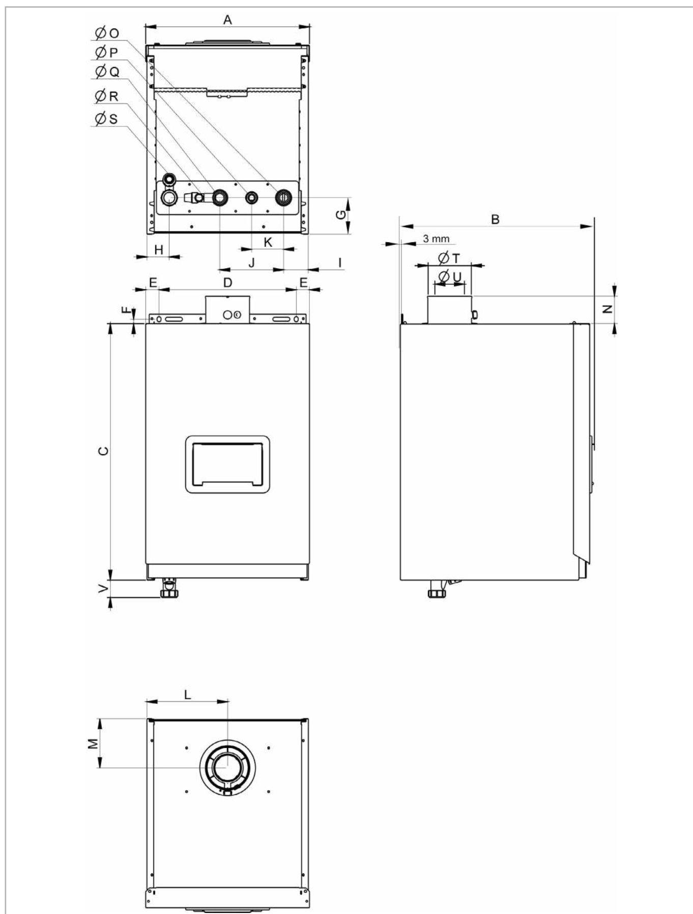
figura 1 - Caratteristiche dimensionali
