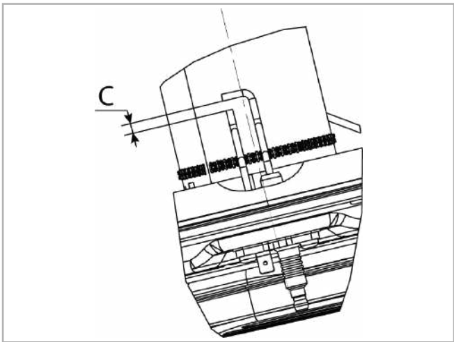
figura 25 - Geometria elettrodo
