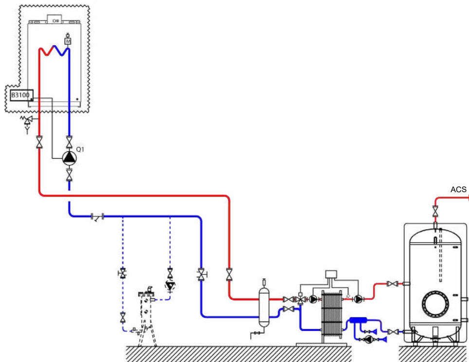
figura 32 - Schema VARFREE EVO22
