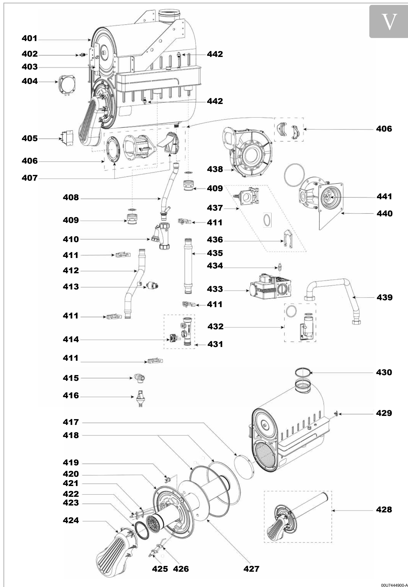
figura 45 - Corpo e bruciatore modello 150 kW
