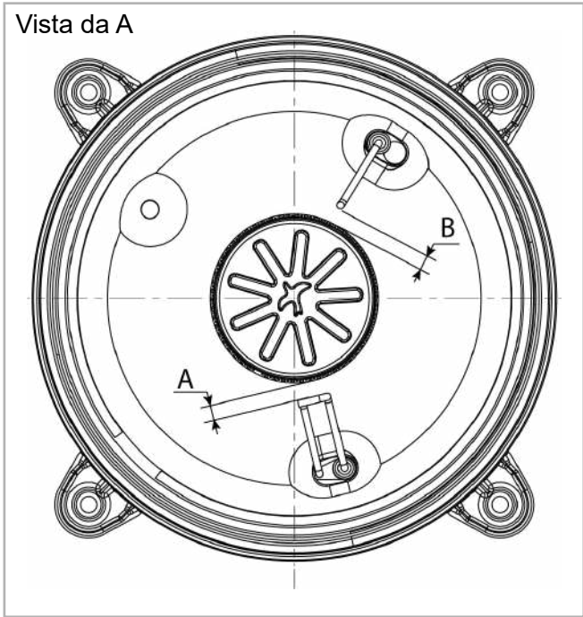
figura 24 - Posizione elettrodi bruciatore
