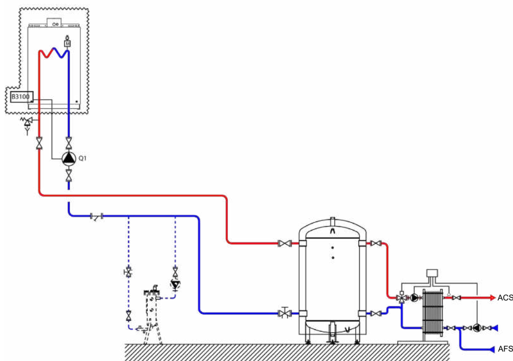
figura 33 - Schema VARFREE EVO23
