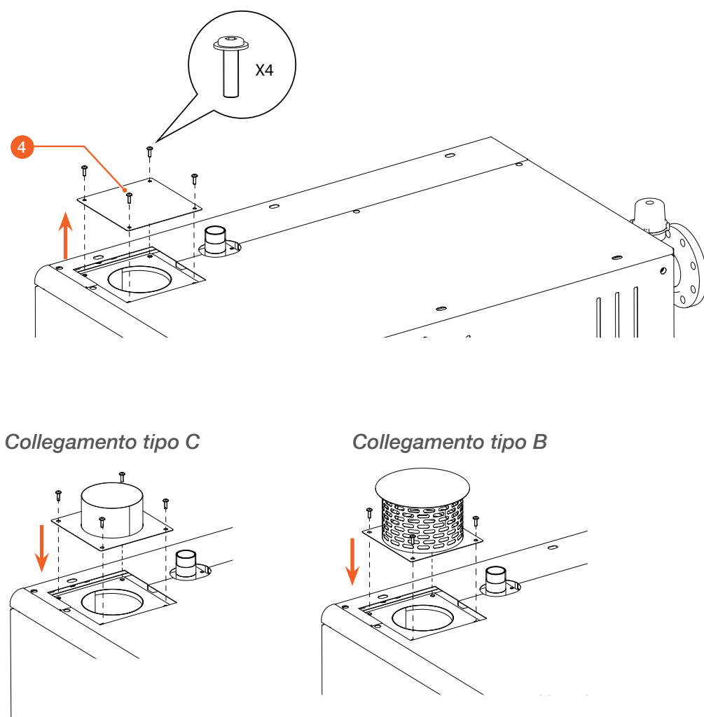
Fig. 15. Installazione ingresso aria
