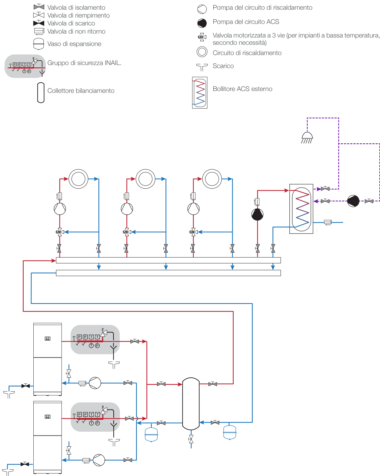
Fig. 20. Caldaie in cascata, con bollitore esterno per acqua calda sanitaria e collettore bilanciamento
