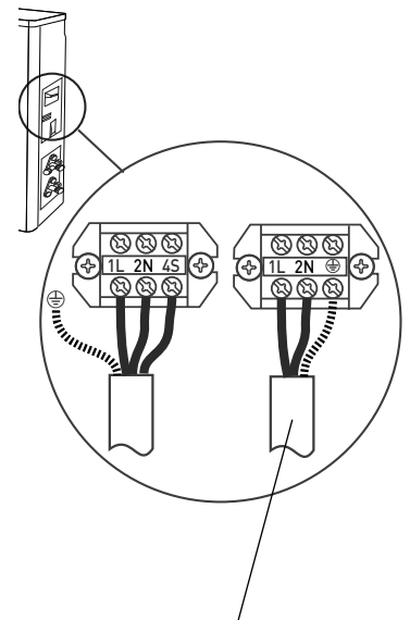
ELEKTRICITEITSNET (H07RN-F)
