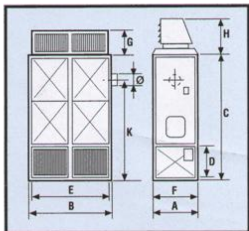
Testata pluridirezionale di distribuzione aria.
