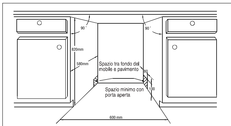
Dimensioni del vano Meno di 5 mm fra la sommità della lavastoviglie e del vano e la porta esterna allineata al vano
