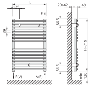
16 Tubi
