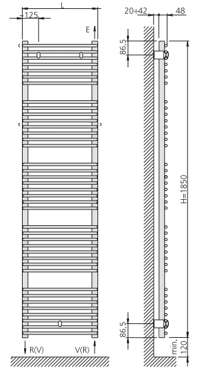
39 Tubi
