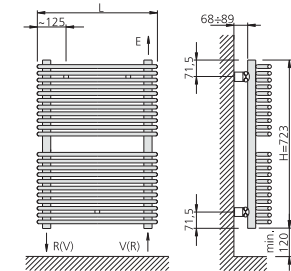
22 Tubi
