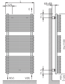
33 Tubi
