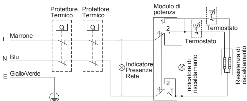
Schema elettrico
