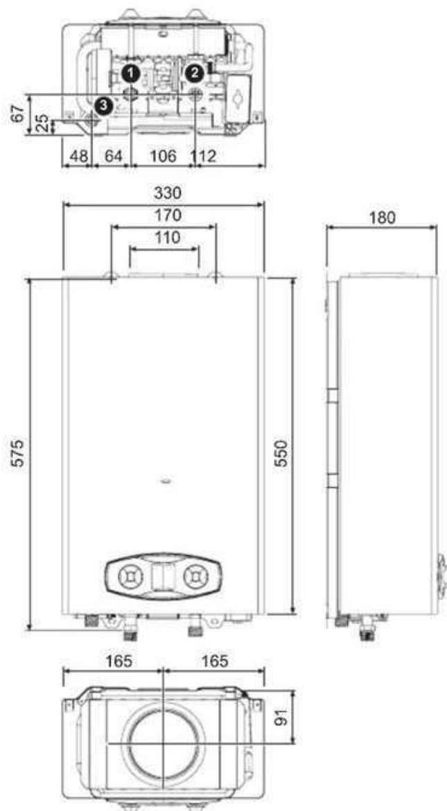
fig. 20 - Dimensiuni și racorduri ZEFIRO ECO 11
