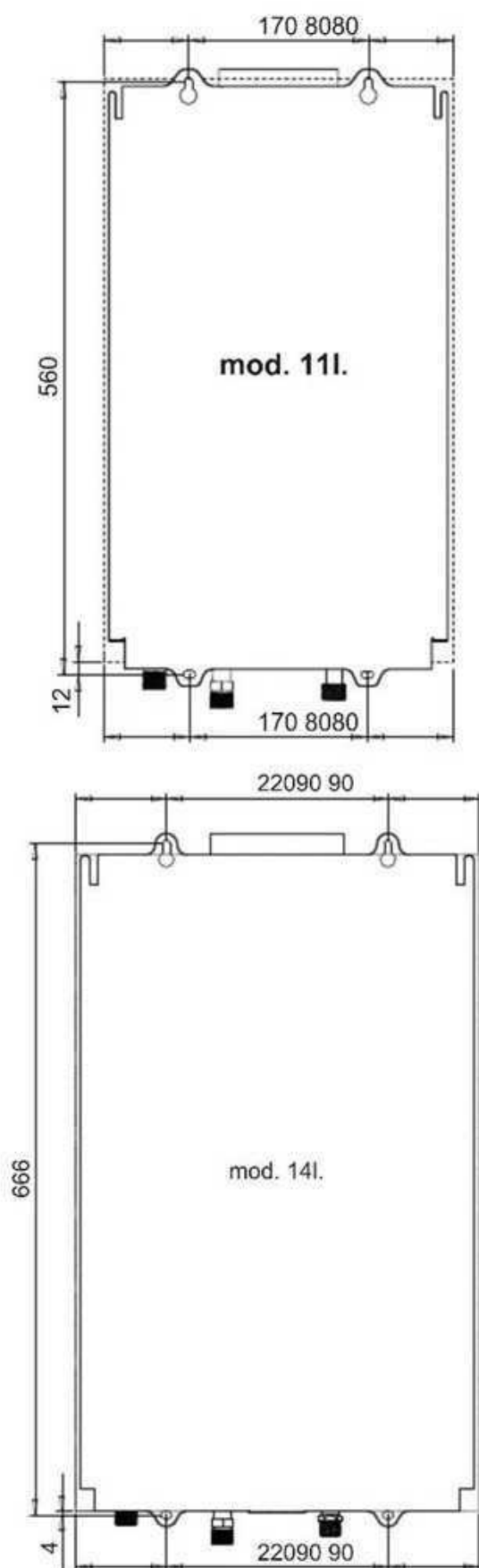
fig. 6 - Assembly template
