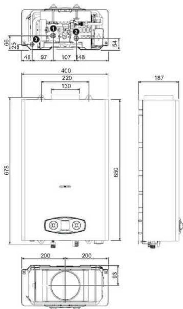
fig. 21 - Dimensioni și racorduri ZEFIRO ECO 14
