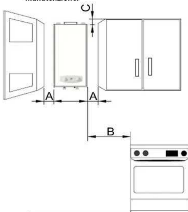
fig. 5 - Distanze minime
