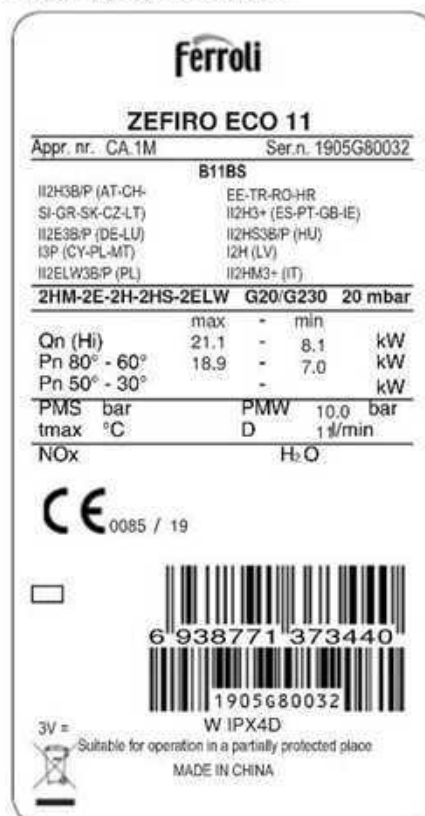
fig. 7 - Tabliczka znamionowa
