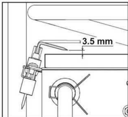
fig. 16 - Posizione elettrodo
