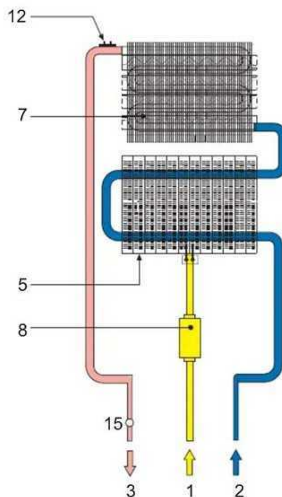
fig. 25 - Circuito idraulico
