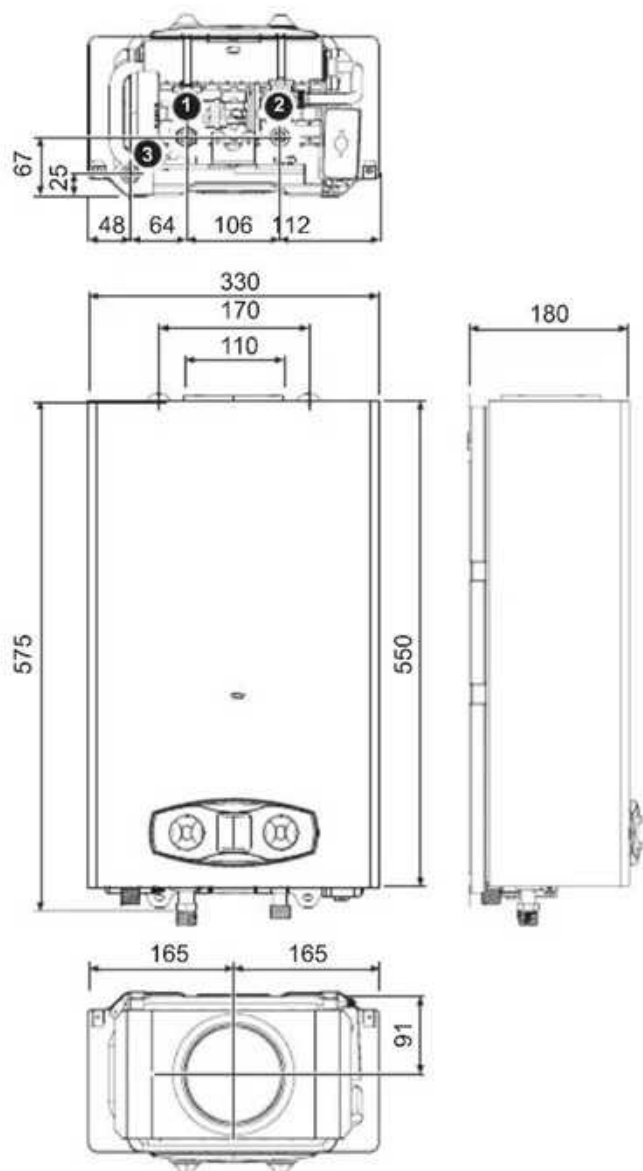
fig. 20 - Dimensioni e attacchi ZEFIRO ECO 11
