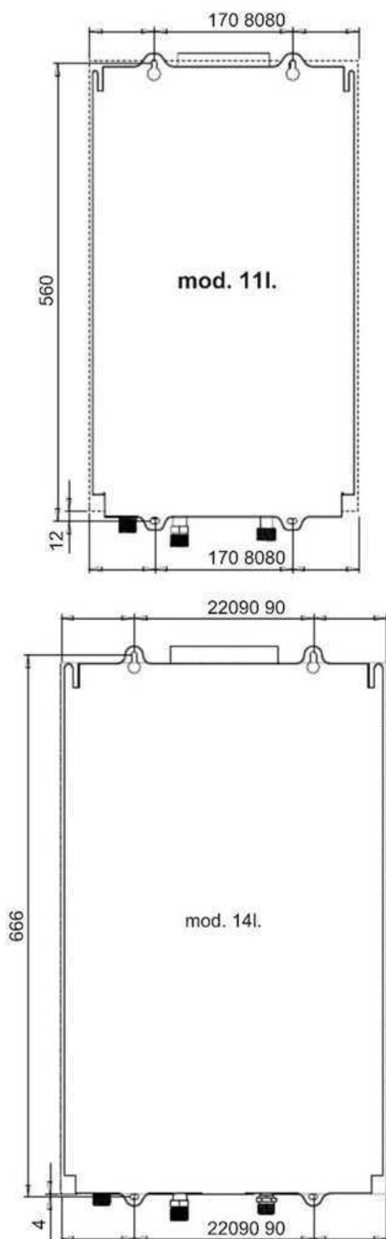
fig. 6 - Szablon montażowy
