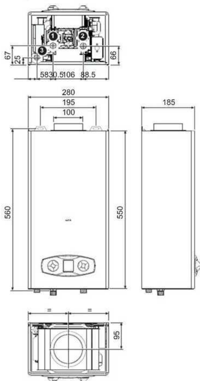
fig. 20 - Wymiary i podłączenia ZEFIRO ECO 6
