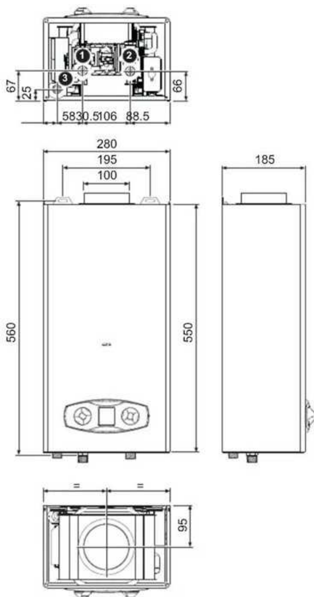
fig. 19 - Dimensioni e attacchi ZEFIRO ECO 6
