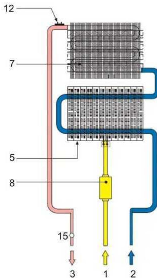
fig. 26 - Obwód hydrauliczny
