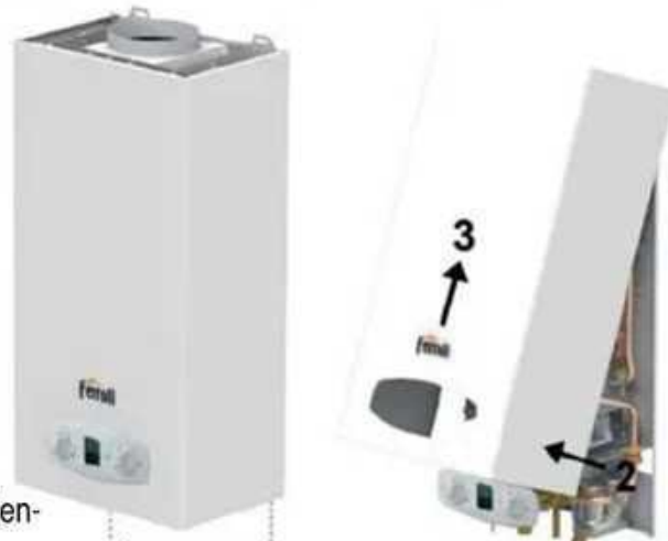
fig. 17 - Otwarcie obudowy
