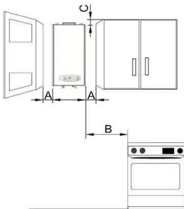
fig. 5 - Distanțe minime
