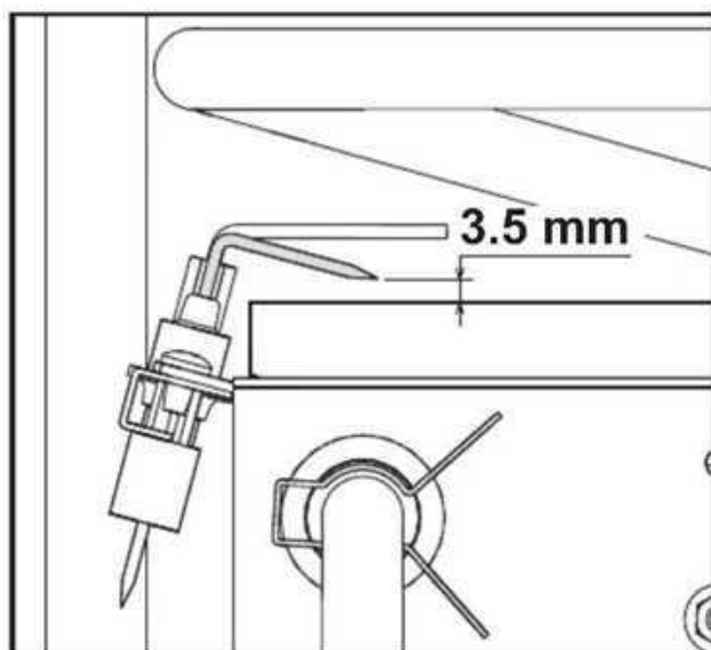
fig. 16 - Poziție electrozi
