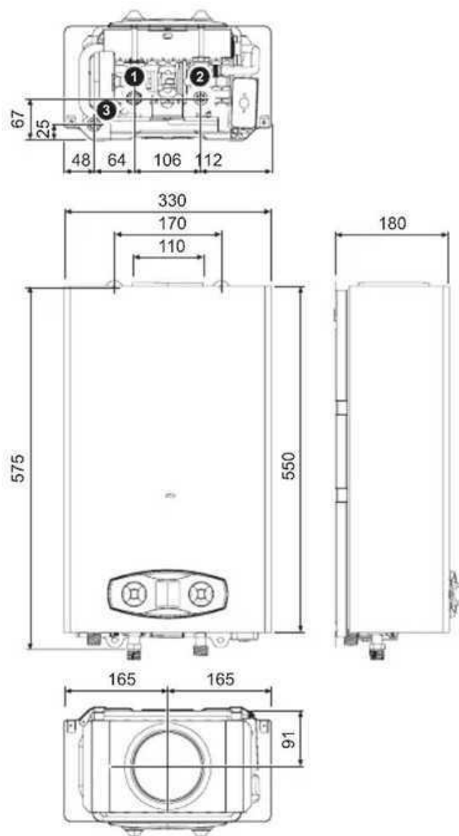
fig. 21 - Wymiary i podłączenia ZEFIRO ECO 11
