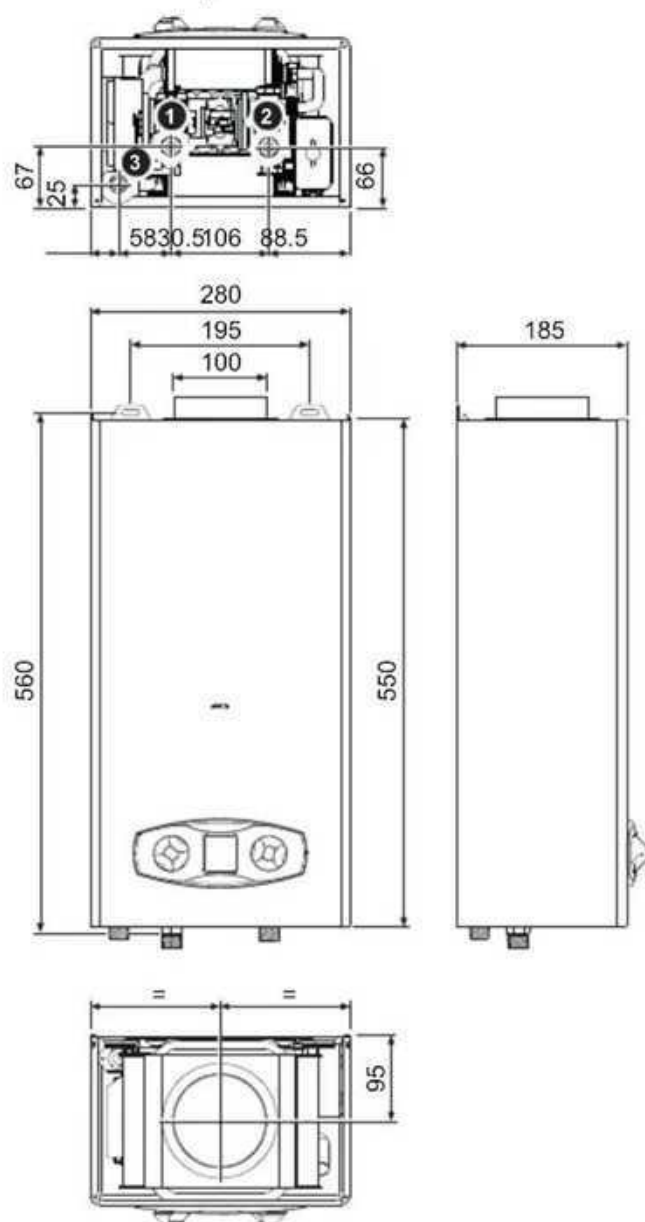
fig. 19 - Dimensiuni și racorduri ZEFIRO ECO 6
