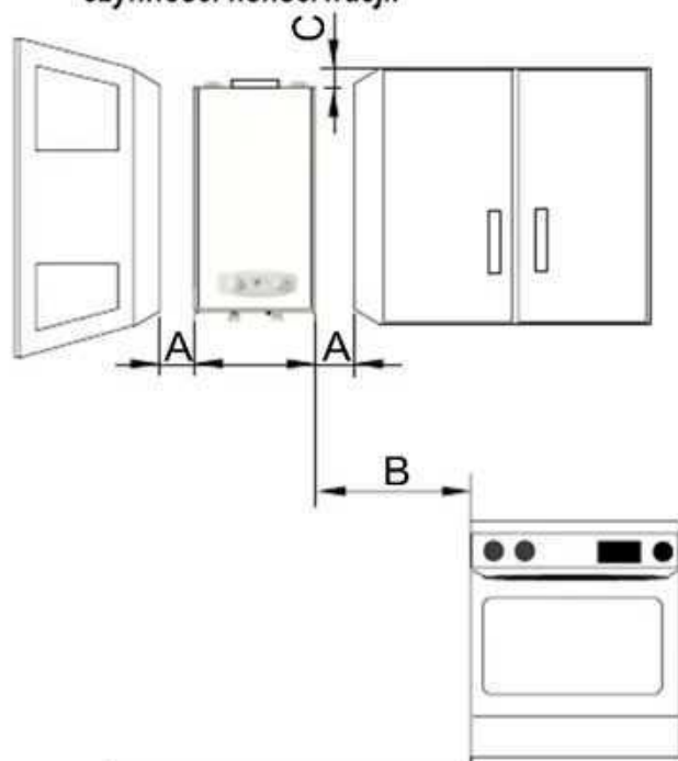
fig. 5 - Minimalne odległości
