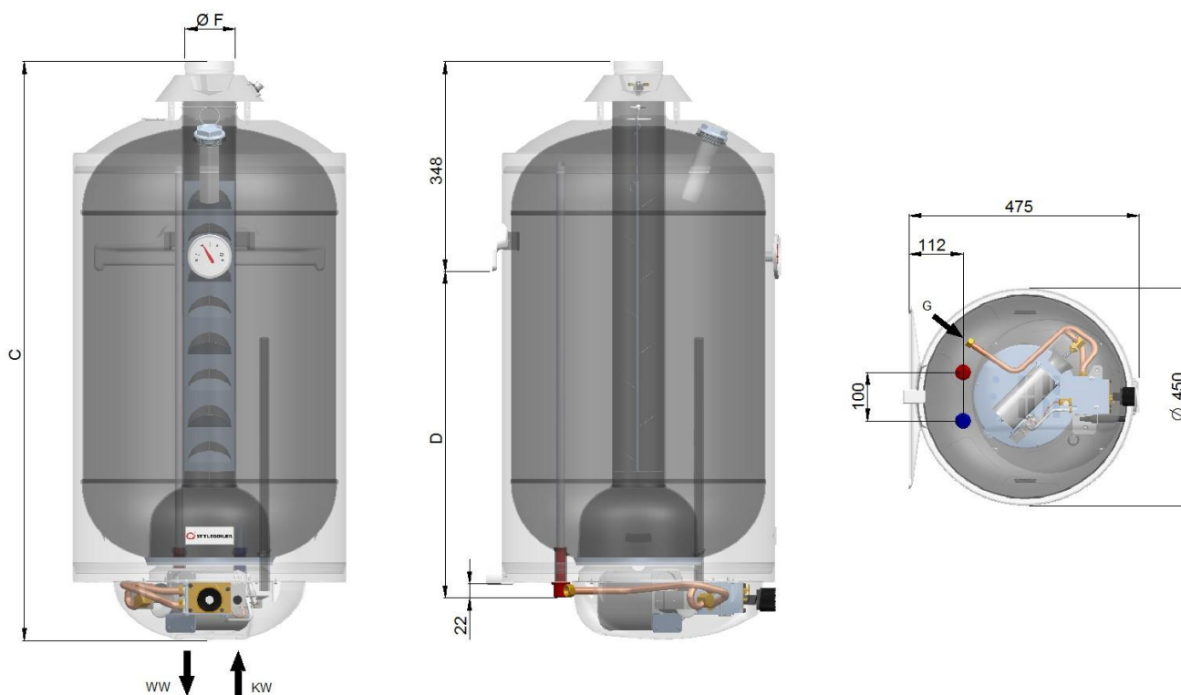
FIGURA 1 – DIMENSIONI SERIE 100-120
