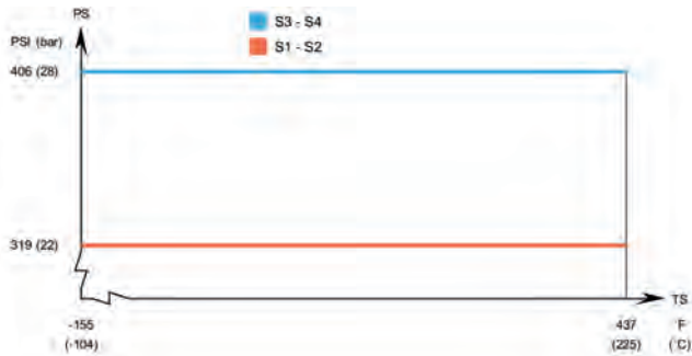
CB300 – Diagramma relativo a temperatura/pressione secondo omologazione UL*
