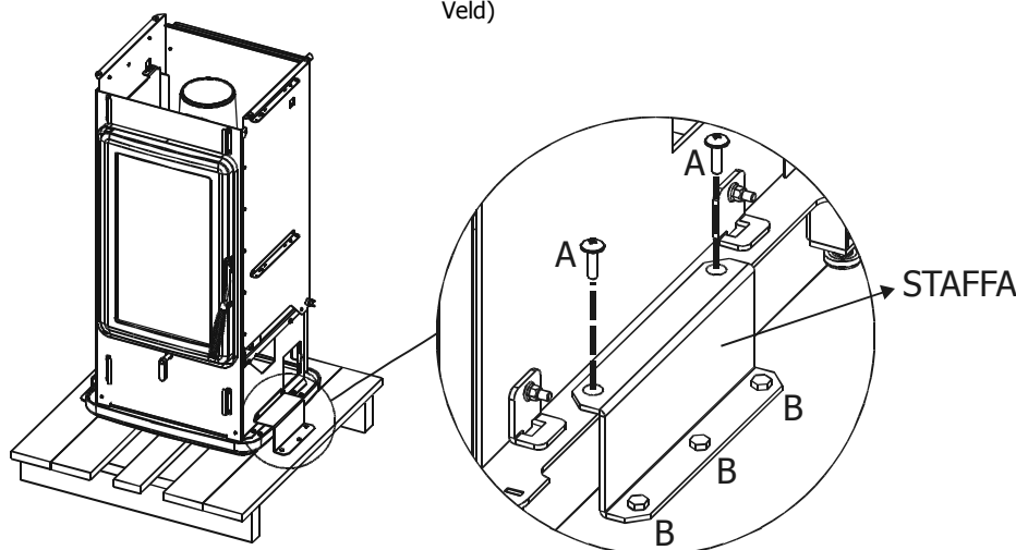
Figura 3 - Rimozione viti imballo (stufa Veld)
