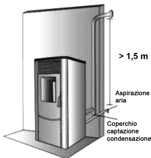
fig 6: installazione di uscita di fumi esterna (SCONSIGLIATA) che si dovrà realizzare di conformità con le norme
