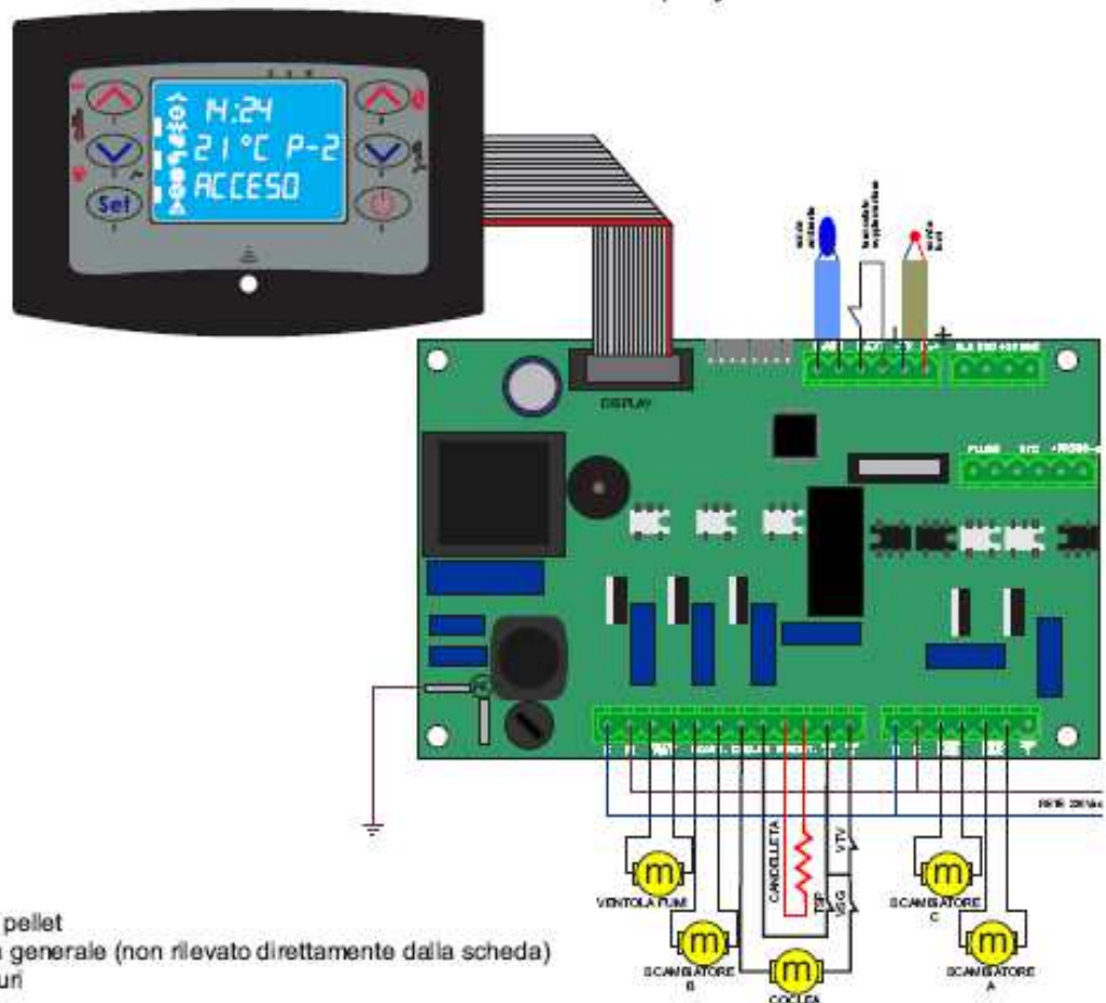
SCHEMA CONNESSIONI M050 aria display evo
