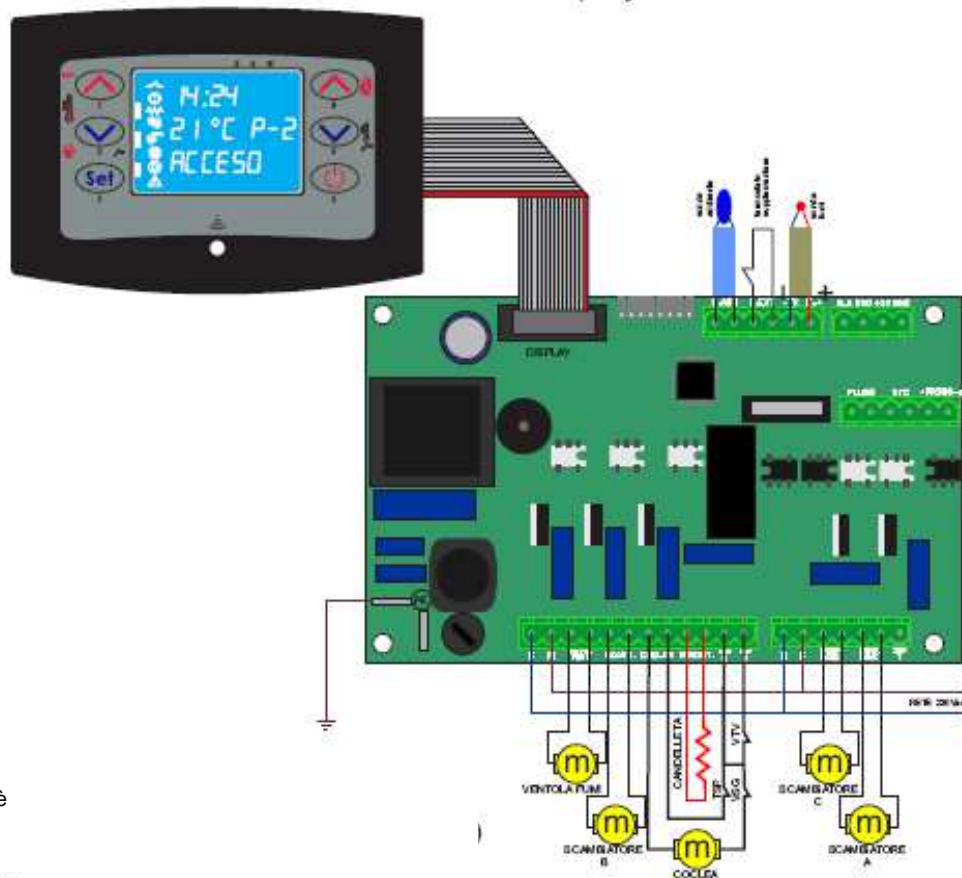
SCHEMA CONNESSIONI M050 aria display evo
