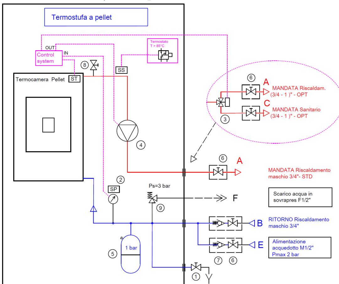
Schema idraulico Termostufa a pellet 10-15 kW_10-2015
