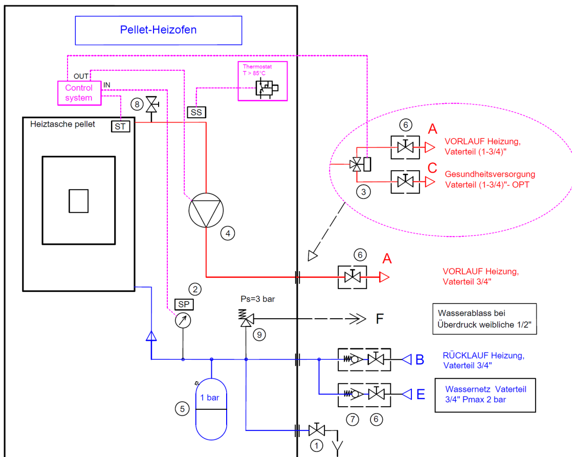
Hydraulischaltplan Pellet-Heizofen 10-15 kW_10-2015
