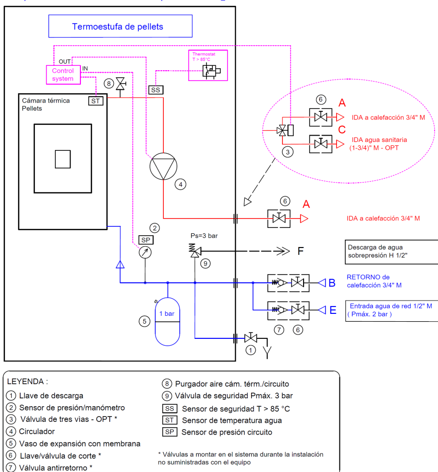
Esquema hidráulico de la termoestufa de pellets 10-15 kW_10-2015
