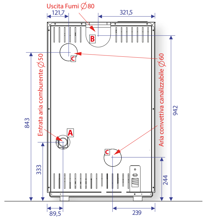
Vista Laterale
