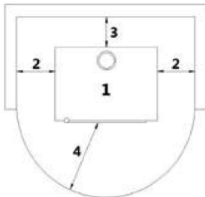
Fig. 15 - Installazione generica
