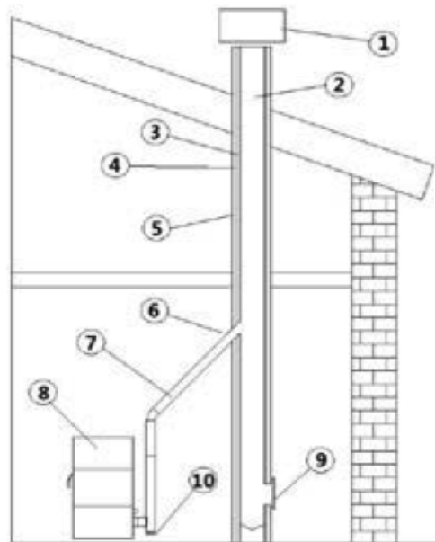
Fig. 5 - Componenti camino
