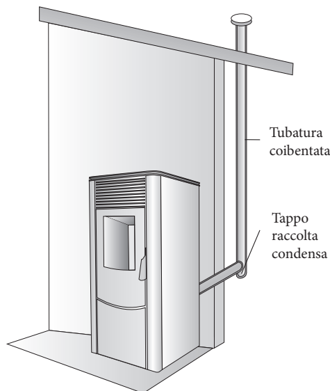
Fig.4: installazione canna fumaria esterna
