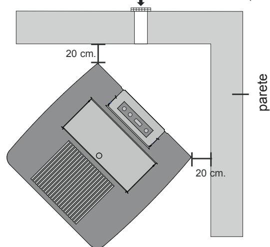
Fig. 9: distanze dai muri entrata aria comburente ( > 120 \text{ cm}^2 )
