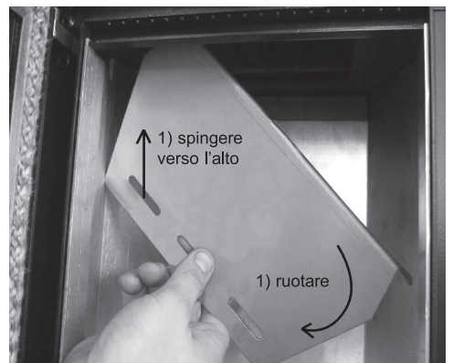
Fig. 14: estrazione del battifiamma
