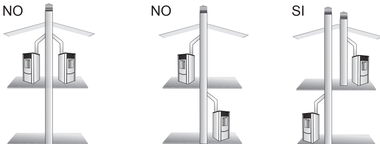
Fig. 1: metodologie d'installazione della canna fumaria
