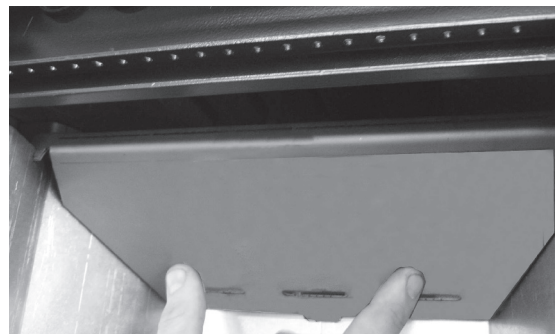
Fig. 14: estrazione del battifiamma
