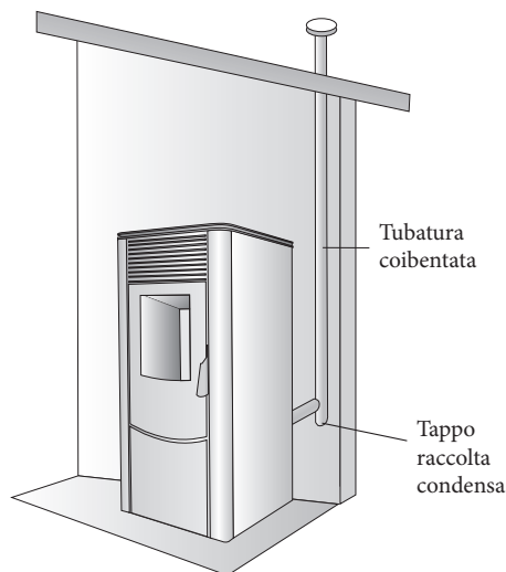
Fig.4: installazione canna fumaria esterna
