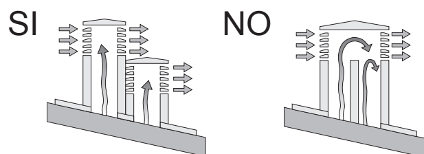
Fig. 2: caratteristiche del comignolo
