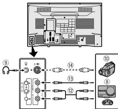
Rückseite des Fernsehgeräts
