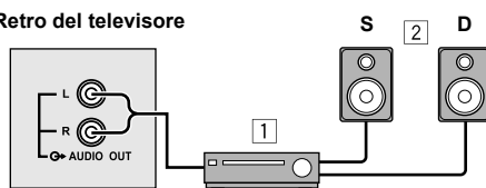
Retro del televisore
