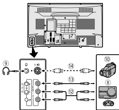
Parte trasera del televisor
