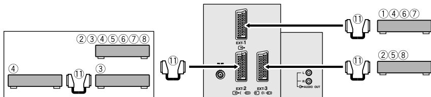
Achterkant van de TV
