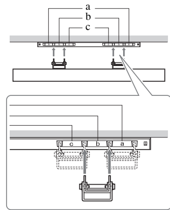
Θέση άγκιστρου
