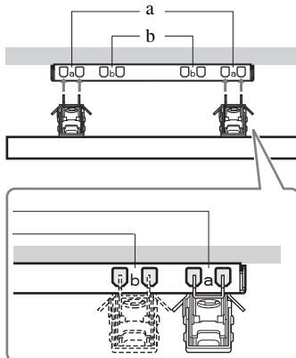
Θέση άγκιστρου
